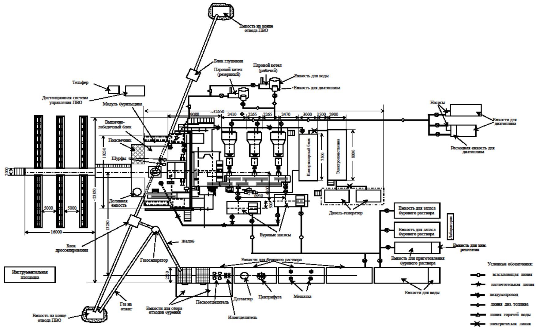
Схема расположения оборудования буровой установки ZJ - 40
