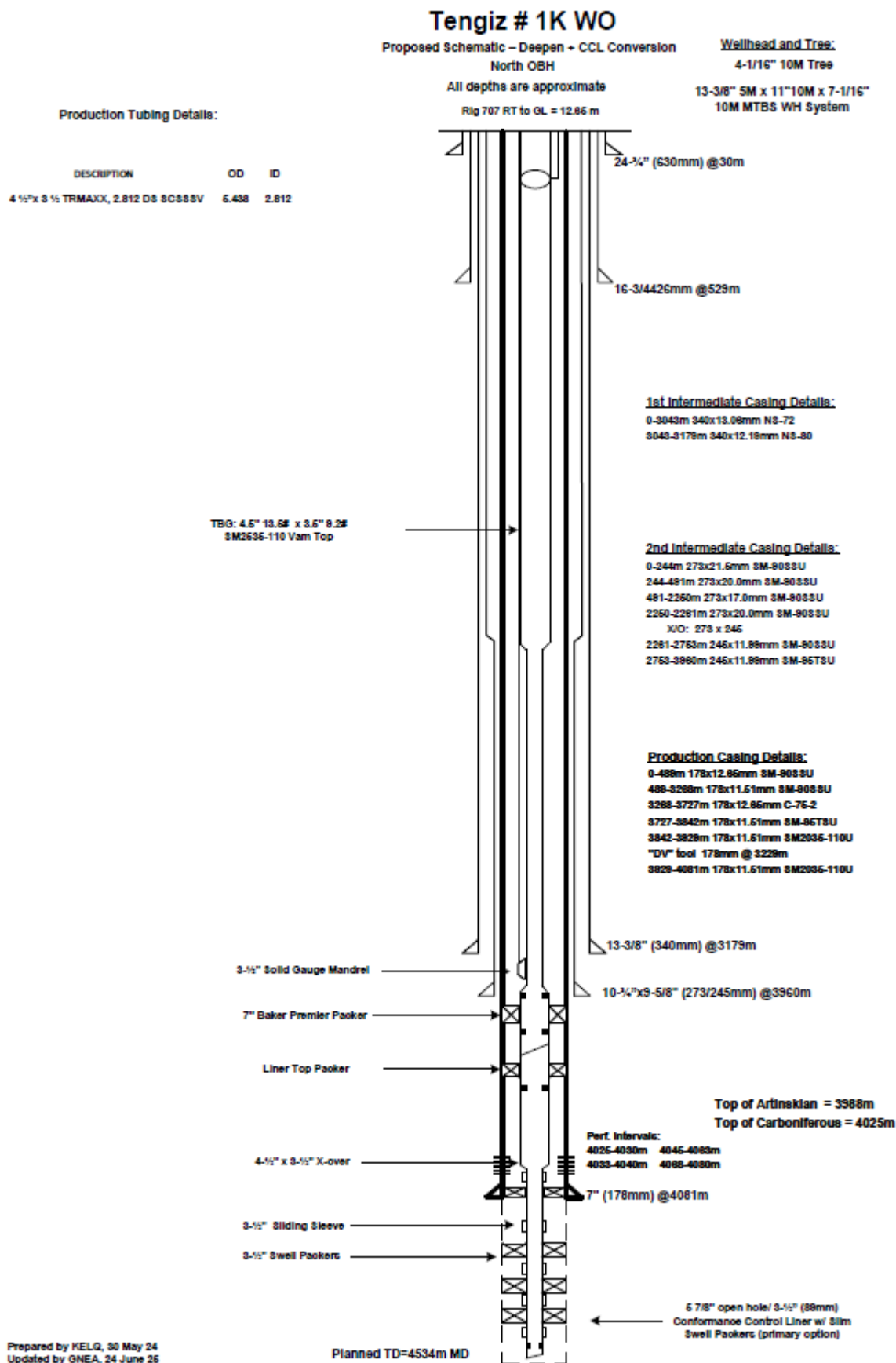
Рисунок 8.1. Скв. Т-0001К Схема ствола скважины
