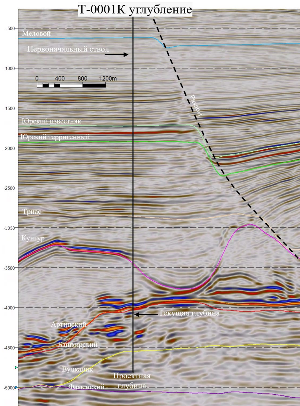
Рисунок 1.4. Сейсмический разрез через скважину Т-0001К
