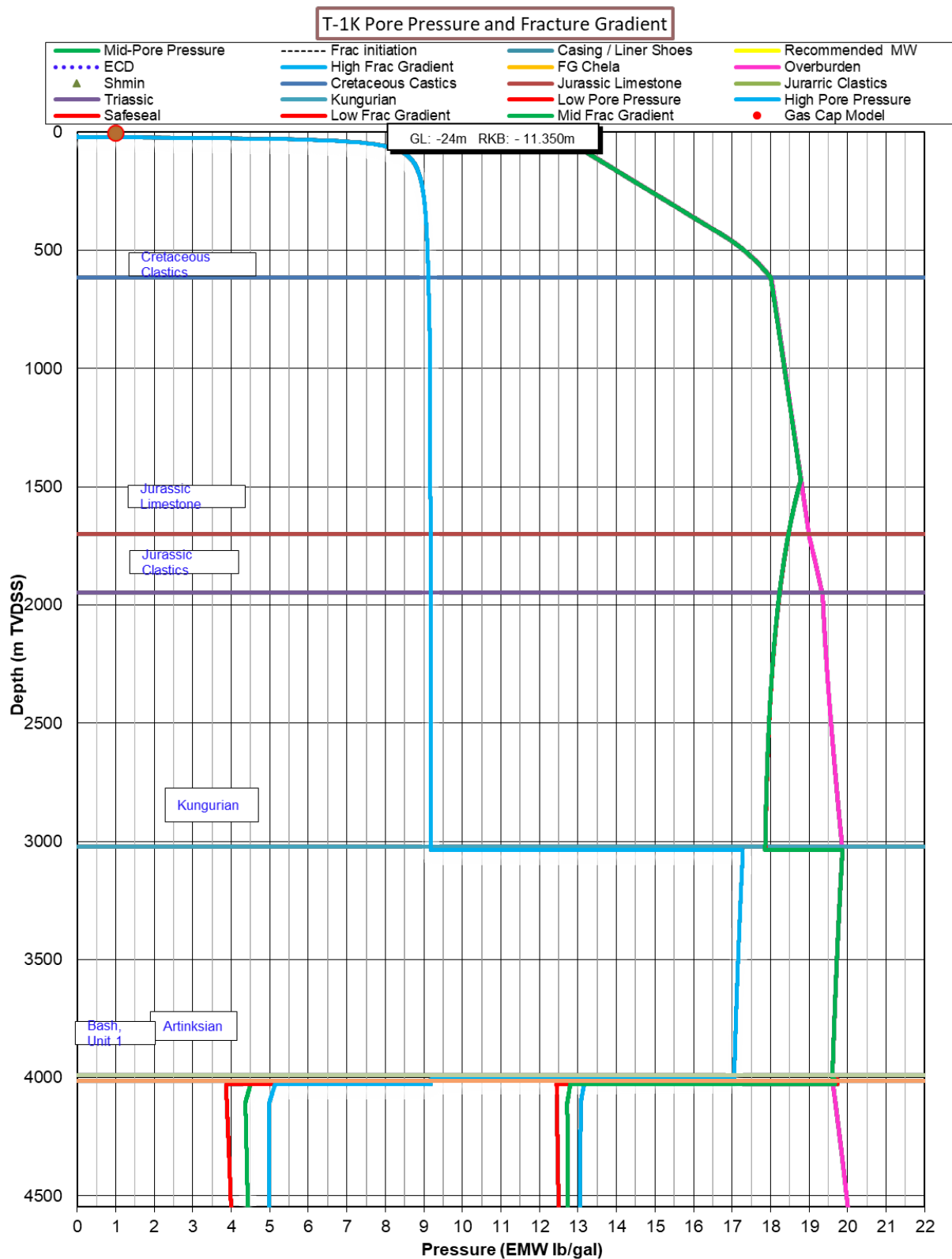
Рисунок 3.1. График совмещенных давлений по колоннам скважины Т-0001К
