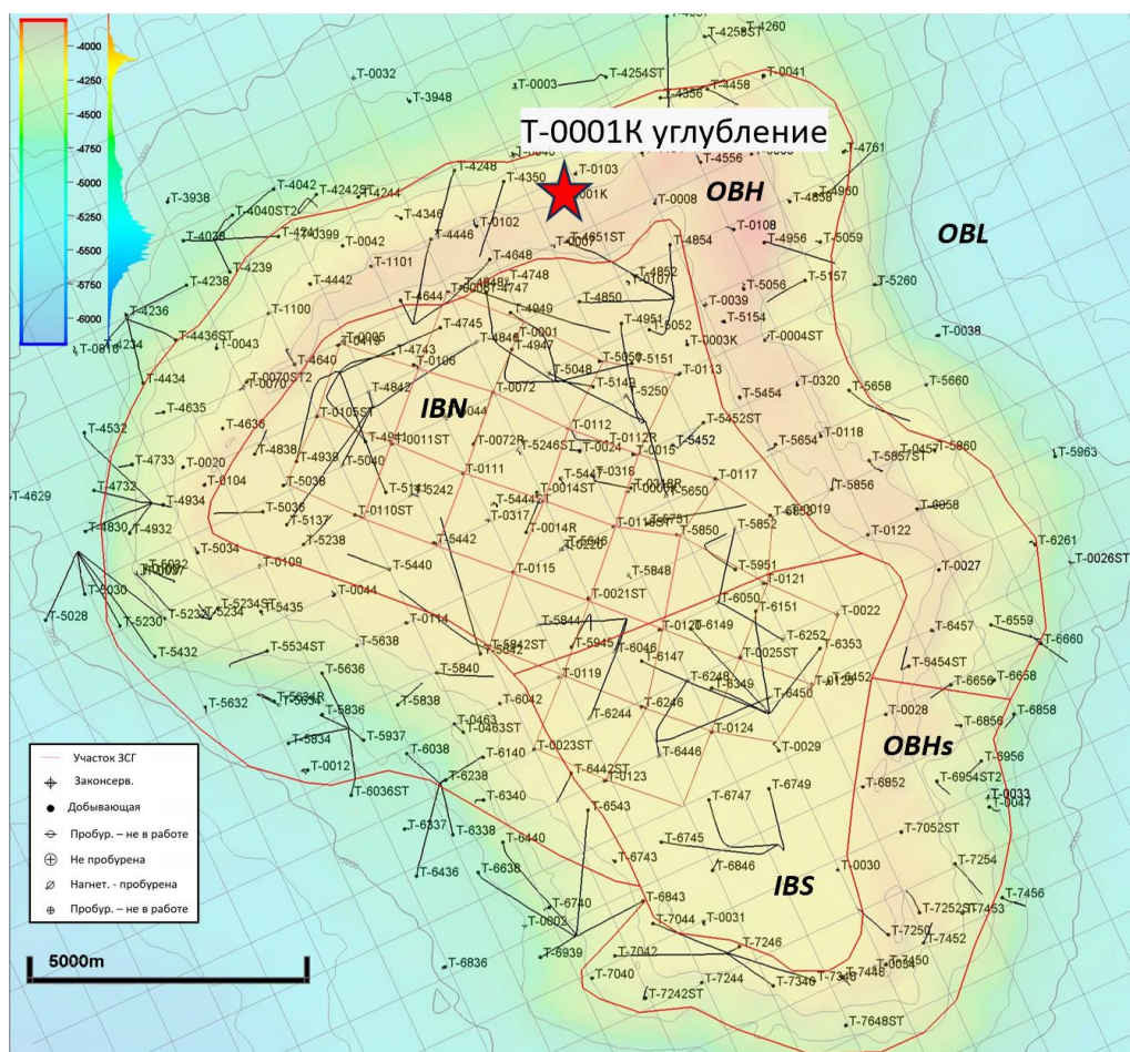
Рисунок 1.2 - Структура кровли коллектора
