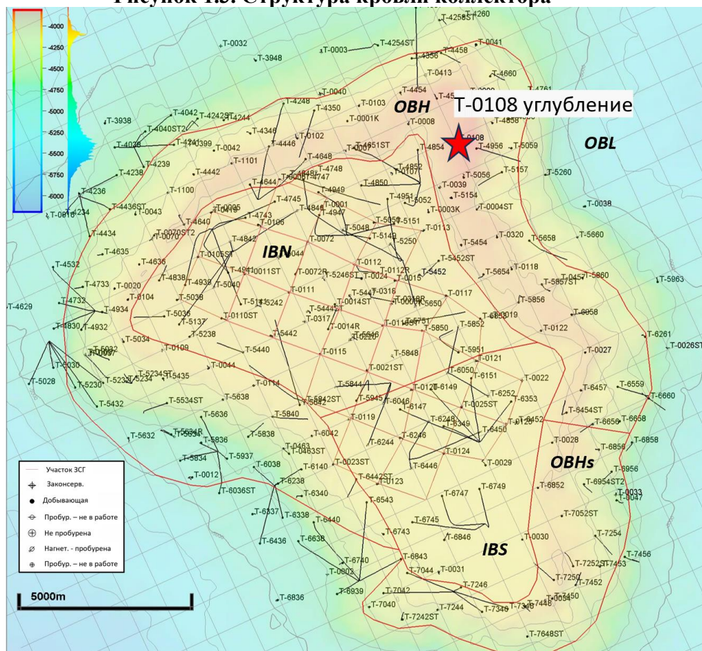
Рисунок 1.3. Структура кровли коллектора
