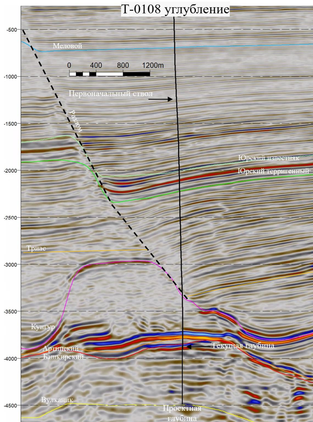
Рисунок 1.4. Сейсмический разрез через скважину Т-0108
