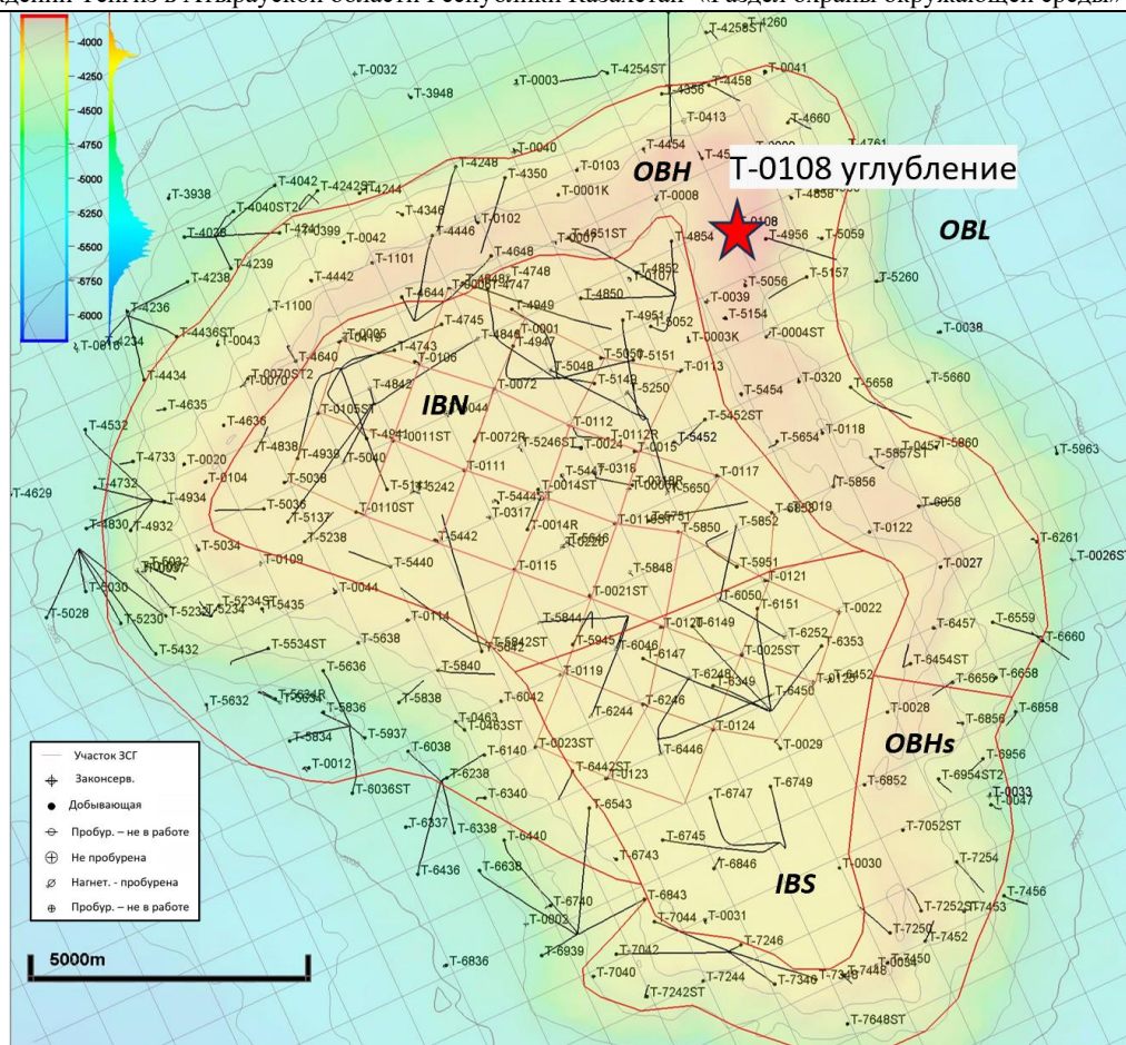
Рисунок 1.2 - Структура кровли коллектора
