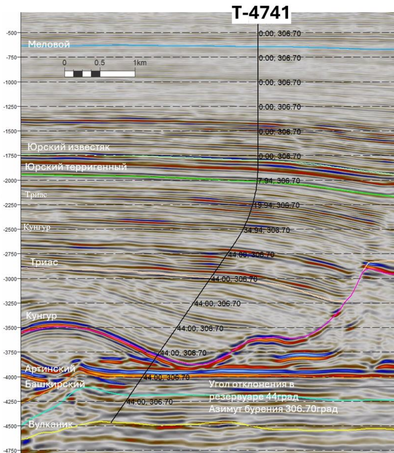
Рисунок 1.4. Сейсмический разрез через скважину Т-4741
