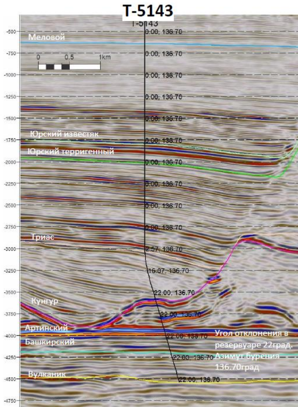
Рисунок 1.4. Сейсмический разрез через скважину Т-5143
