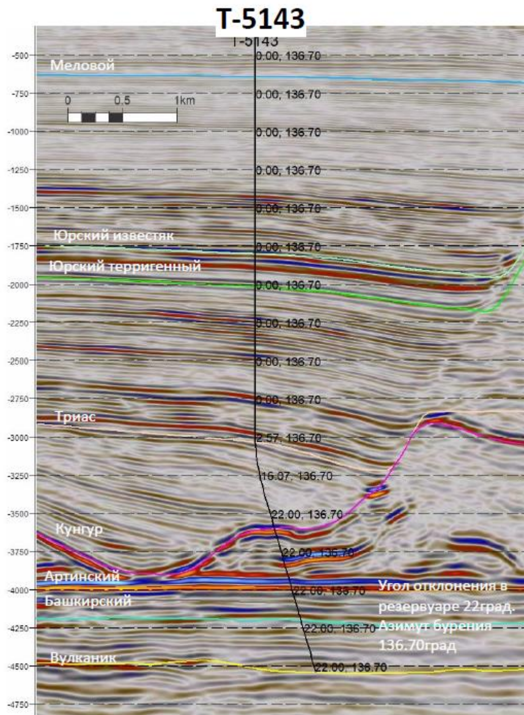
Рисунок 0.2. Сейсмический разрез через скважину Т-5143
