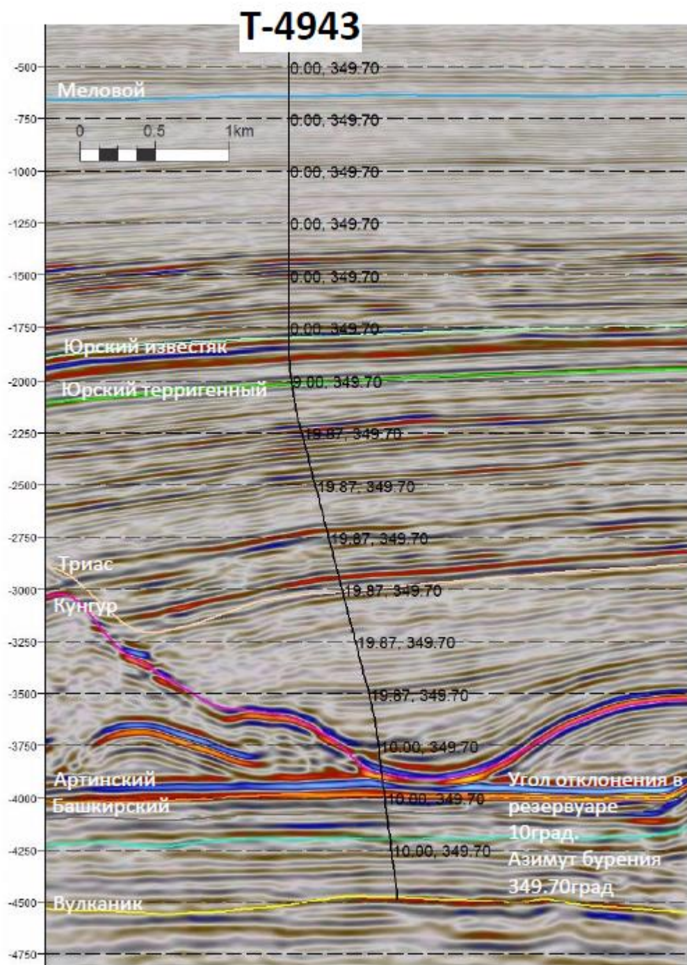
Рисунок 1.4. Сейсмический разрез через скважину Т-4943
