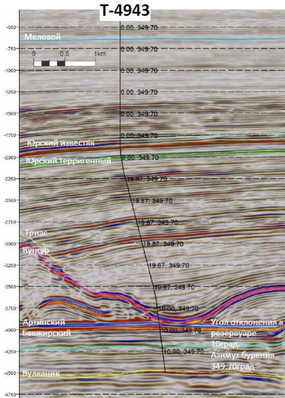
Рисунок 0.2. Сейсмический разрез через скважину Т-4943
