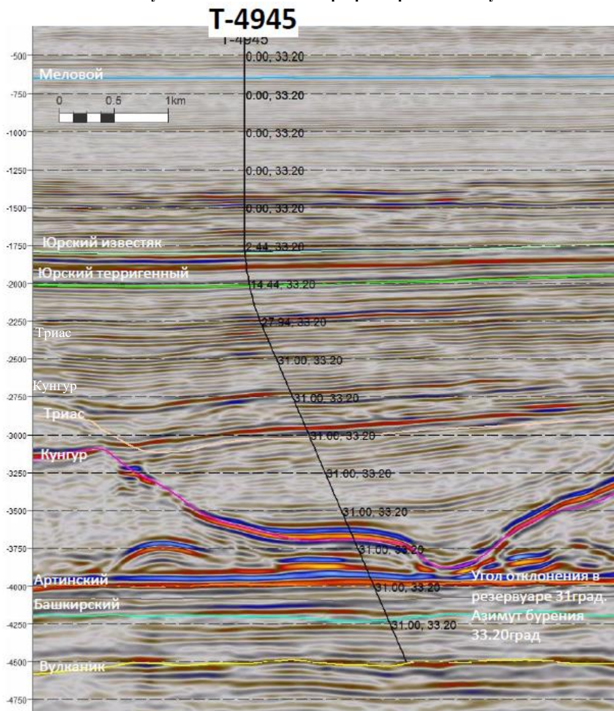
Рисунок 1.4. Сейсмический разрез через скважину Т-4945
