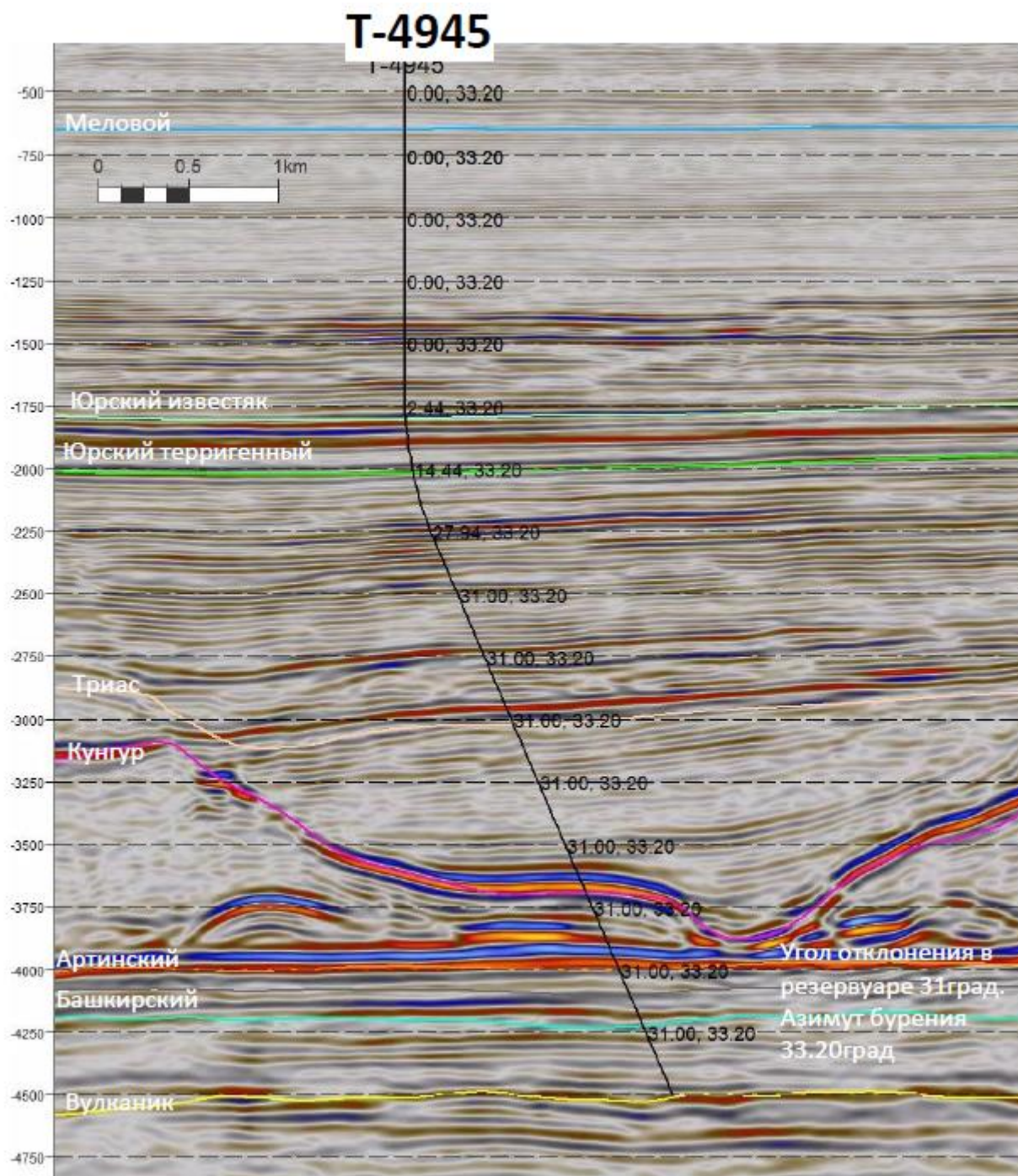
Рисунок 0.2. Сейсмический разрез через скважину Т-4945
