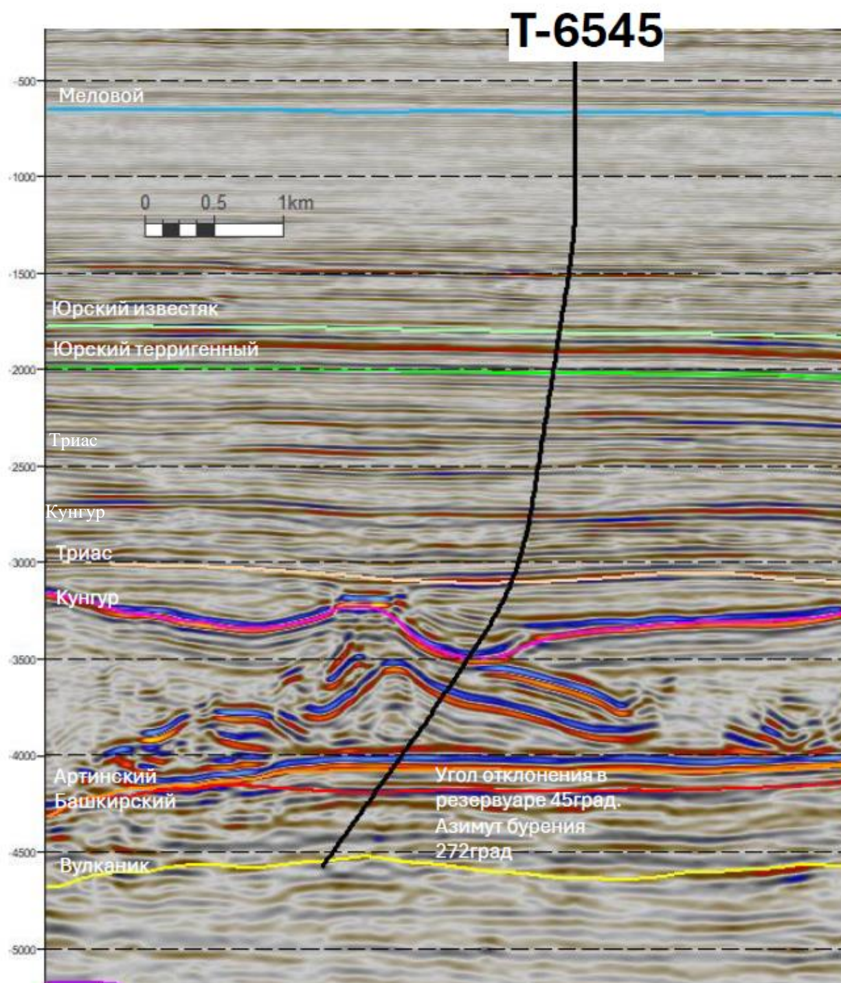
Рисунок 1.4. Сейсмический разрез через скважину Т-6545
