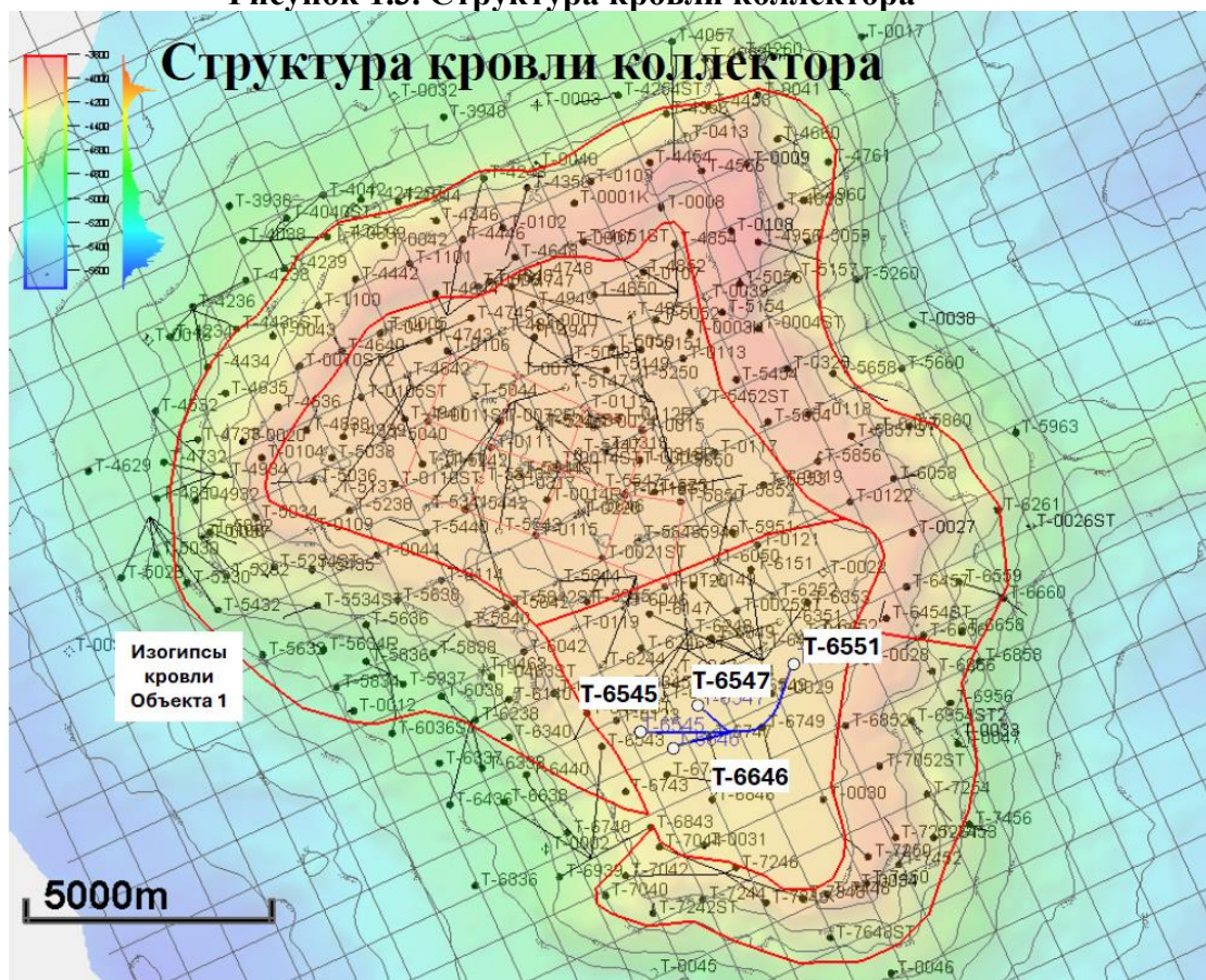
Рисунок 1.3. Структура кровли коллектора
