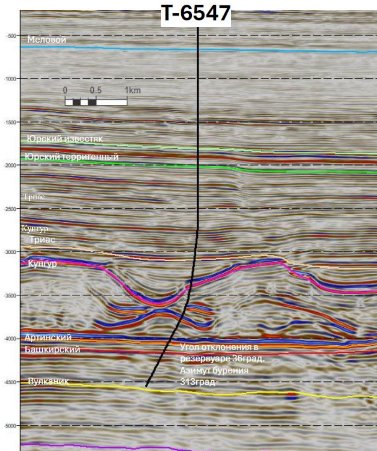
Рисунок 1.4. Сейсмический разрез через скважину Т-6547
