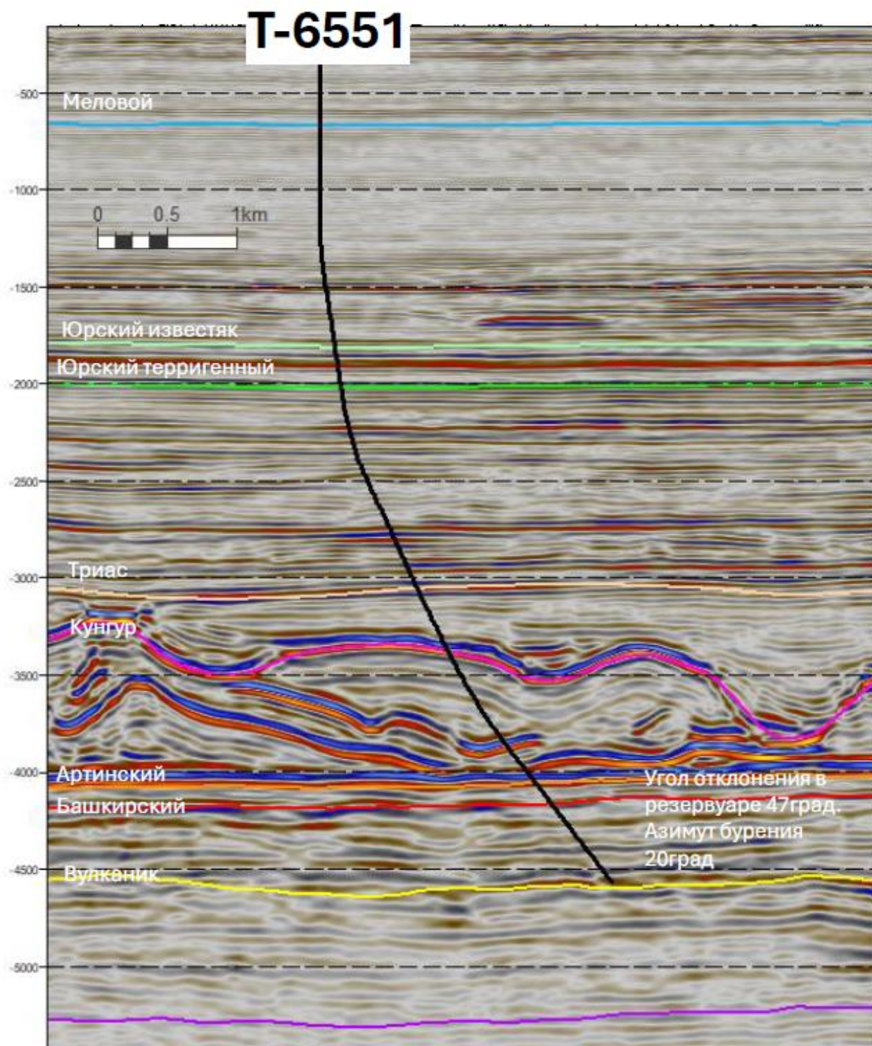
Рисунок 0.2. Сейсмический разрез через скважину Т-6551
