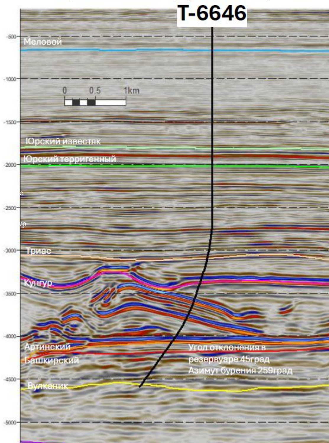
Рисунок 1.4. Сейсмический разрез через скважину Т-6646
