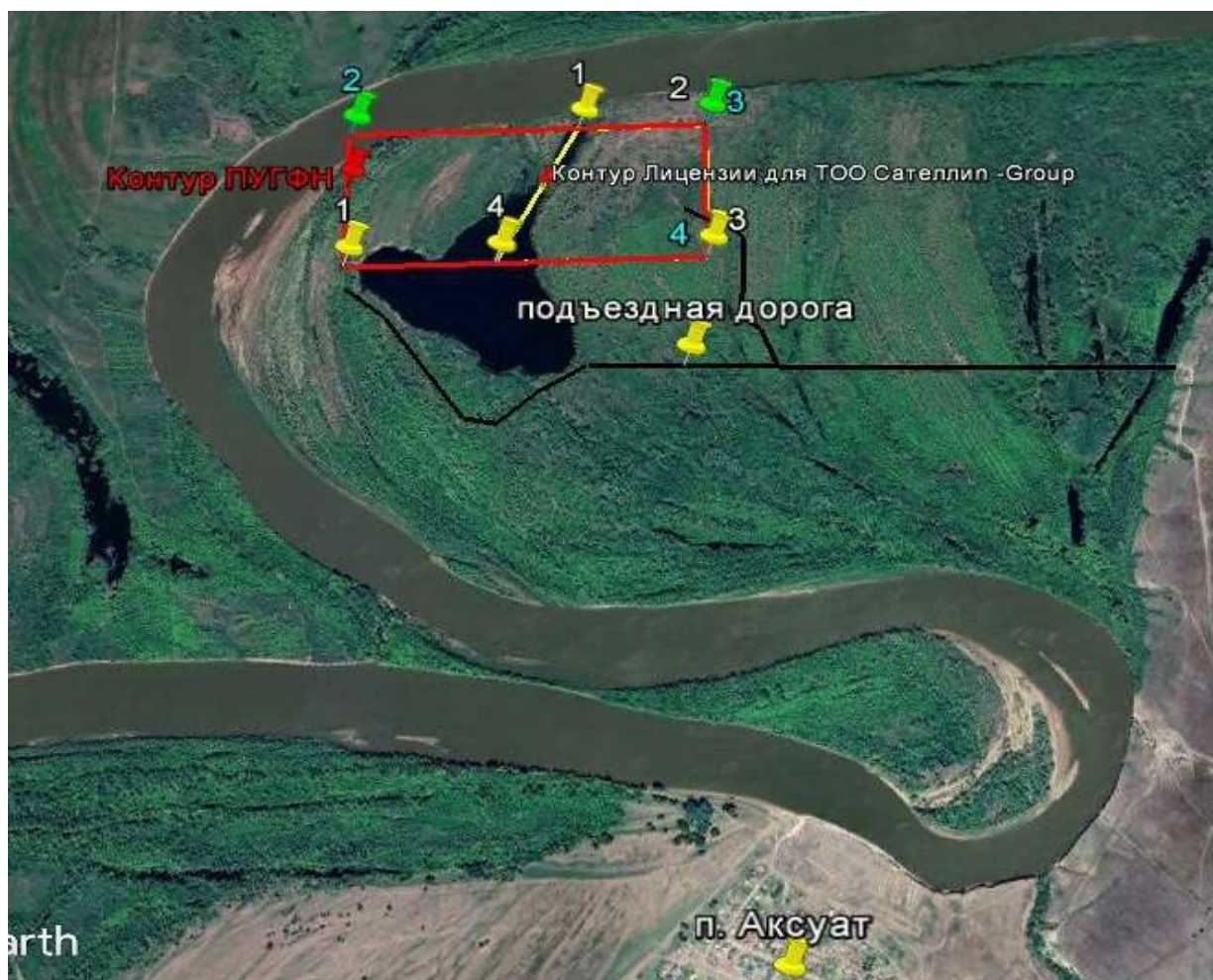
Рис. 4.1.1. Схема расположения Аксуатского месторождения в общей обстановке района
