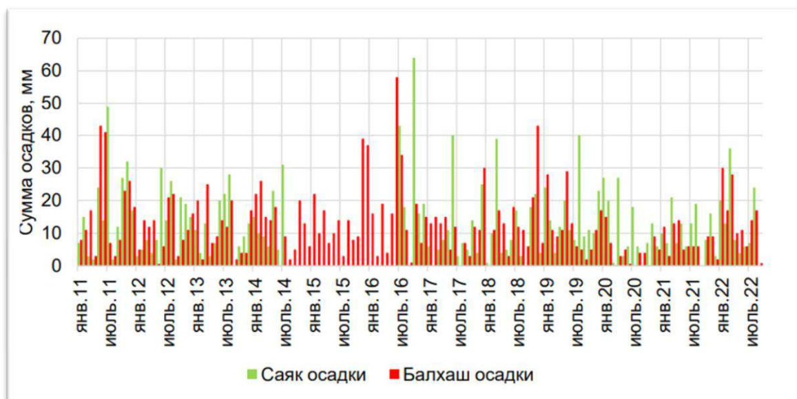
Рисунок 2.2 График суммарных месячных осадков по метеостанции Балхаш и Саяк за 2011–2022 гг.
