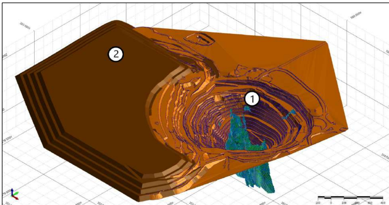
Рисунок 3.1-Месторождение «Пустынное».
