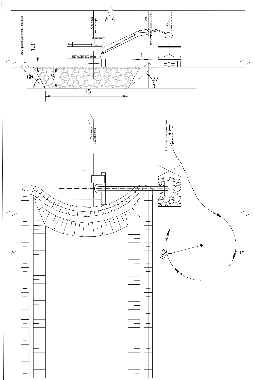
Рисунок 3.4-Схема проходки траншеи (съезда) гидравлическим экскаватором (обратная лопата) с нижним черпанием и погрузкой в автосамосвалы на уровне стояния экскаватора, с петлевым разворотом
