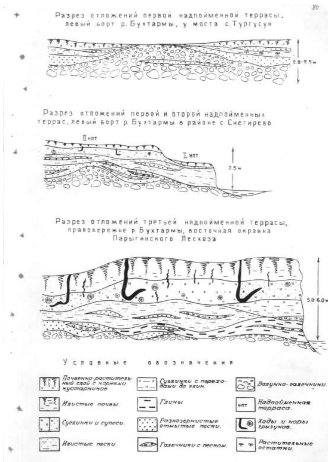
Рис. 2.1 Геологические разрезы
