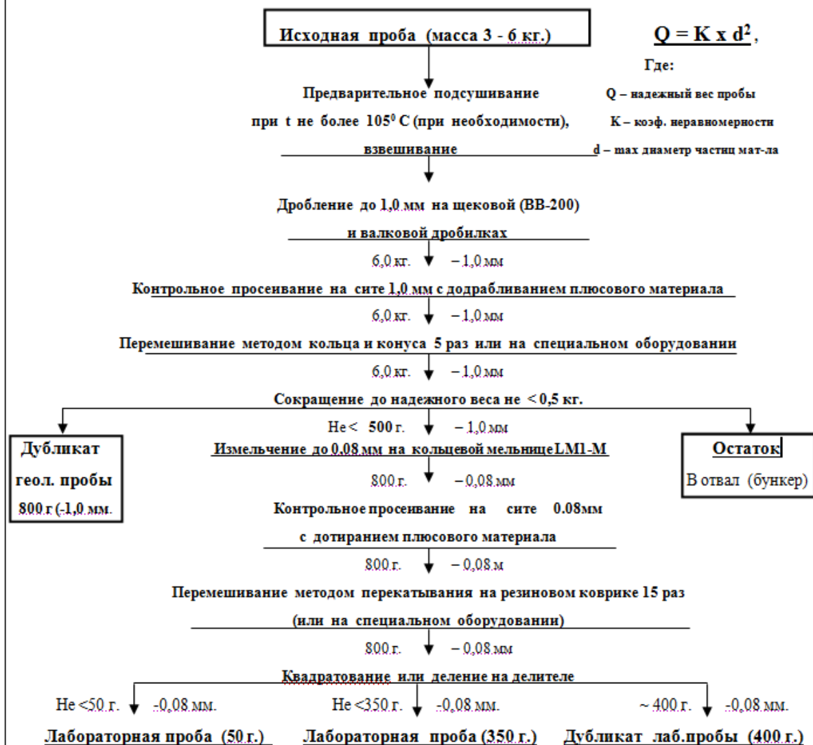
Рис. 3.9.2.1 Схема подготовки kernовых, бороздовых проб весом 3-6 кг
