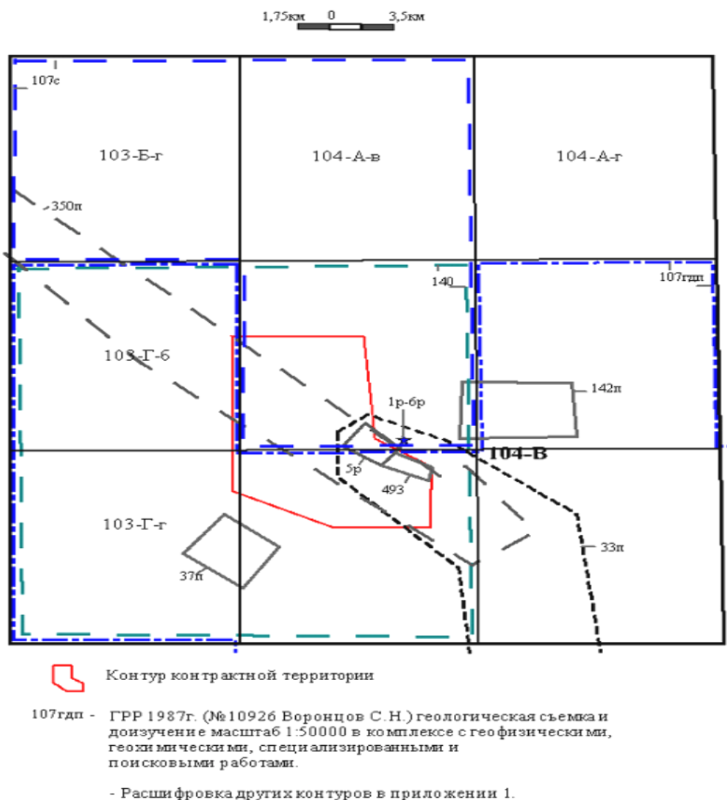
Рисунок 2.1.1 Схематическая картограмма изученности Контрактной территории
