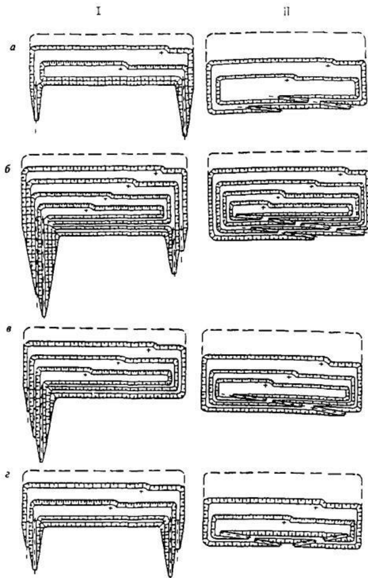
Рис. 2.3. Принципиальная схема способов вскрытия а — отдельными б — групповыми в — общими и г — парными траншеями при внешнем I и внутреннем II заложении траншей
