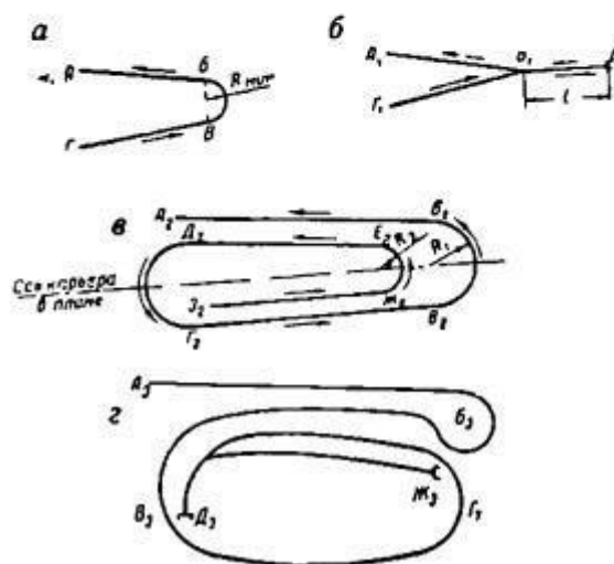
Рис. 2.5. Основные формы плана трассы капитальных траншей а — петлевая б — тупиковая, в — спиральная г — комбинированная, А, Б, В — характерные точки трассы
