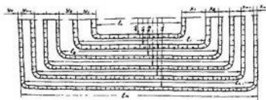
Рис. 2.6. Обозначения исходных данных по карьеру для расчетов вскрытия горизонтов
