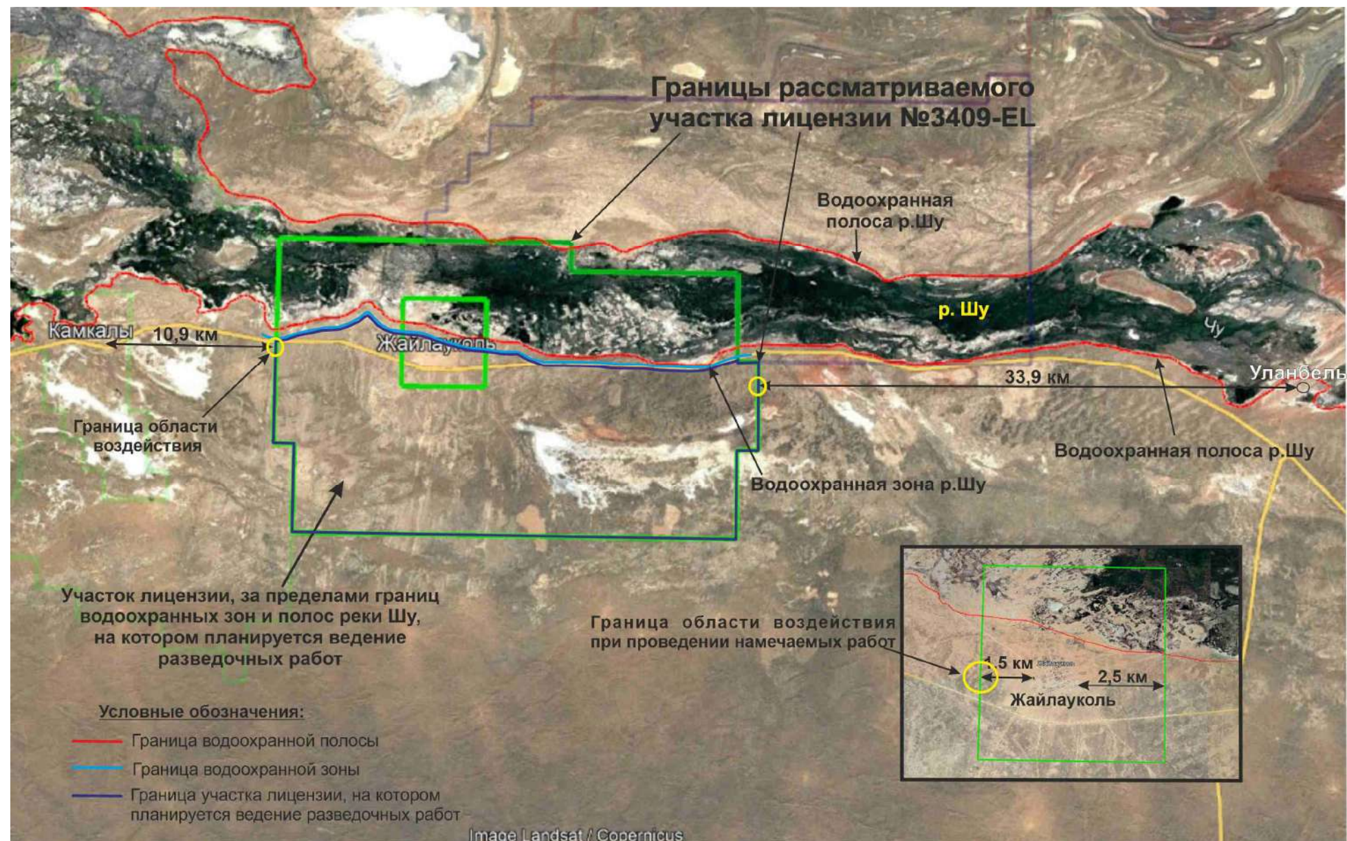
Рисунок 1 – Ситуационная карта-схема района расположения участка лицензии №3409-EL
