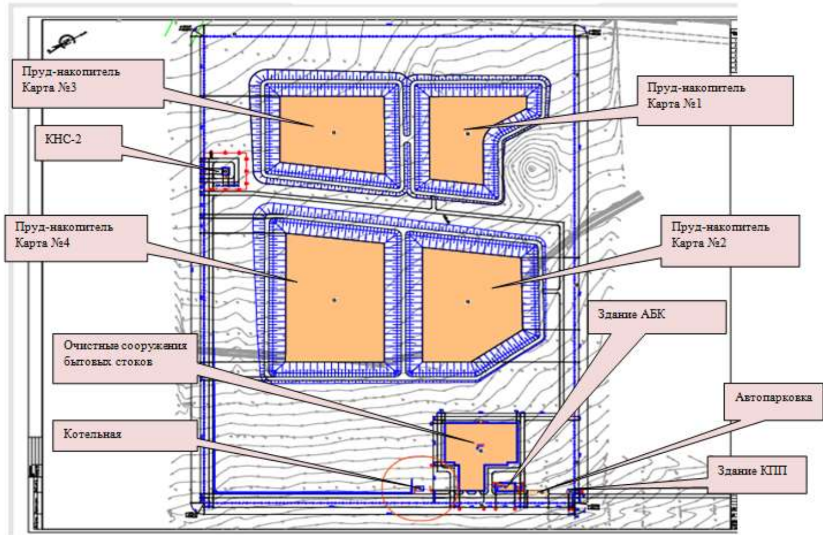
Рисунок 9- Генеральный план КОС
