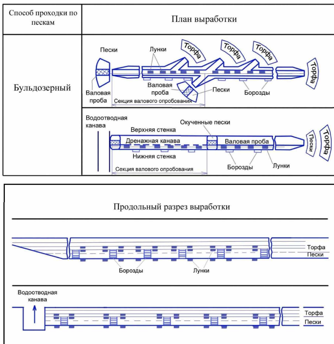
Рис. 5.2 План и продольный разрез проектируемой траншеи
