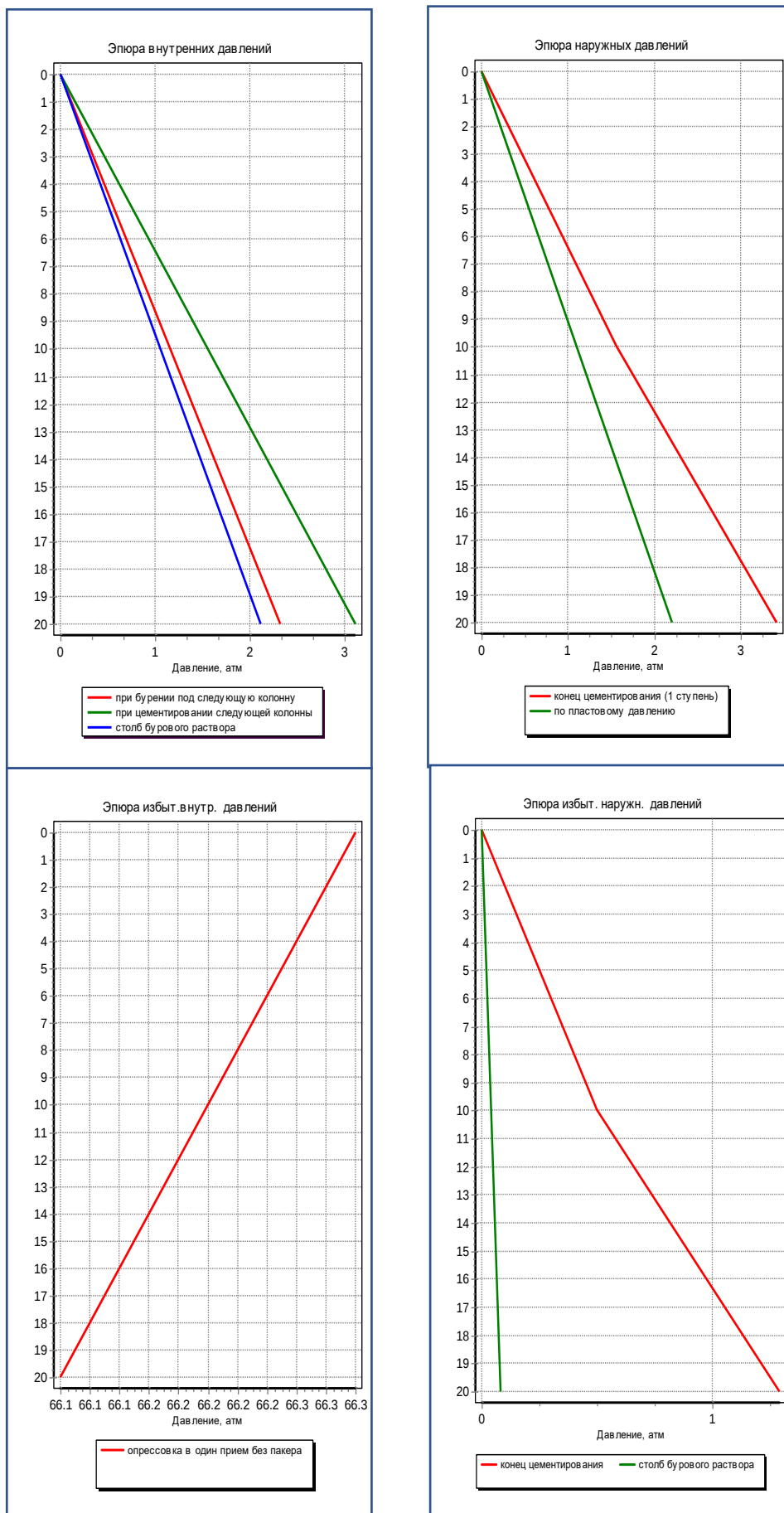
Рисунок 8.1 Направление эпюры давлений
