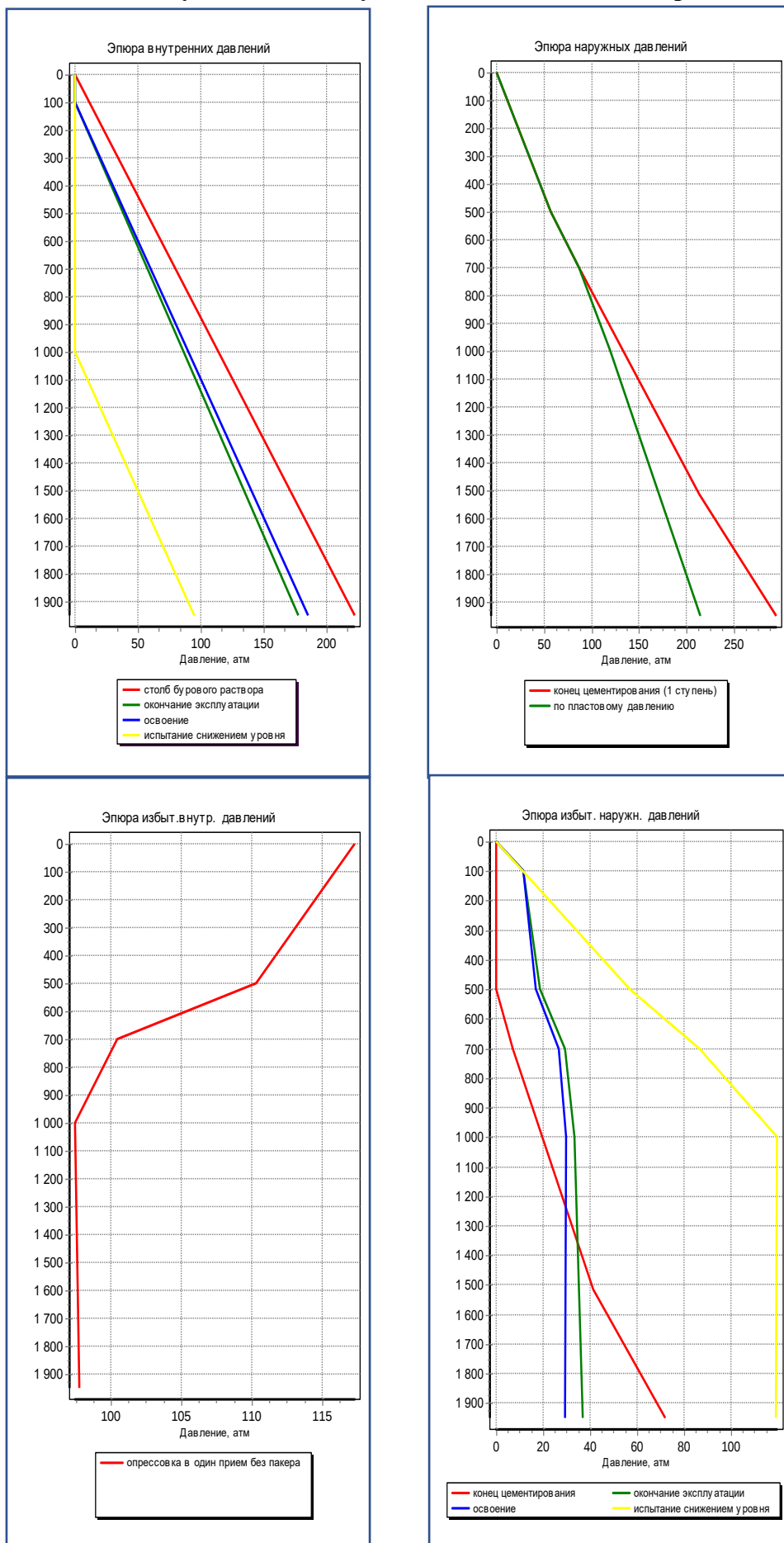
Рисунок 8.4 Эксплуатационная колонна эпюры давлений
