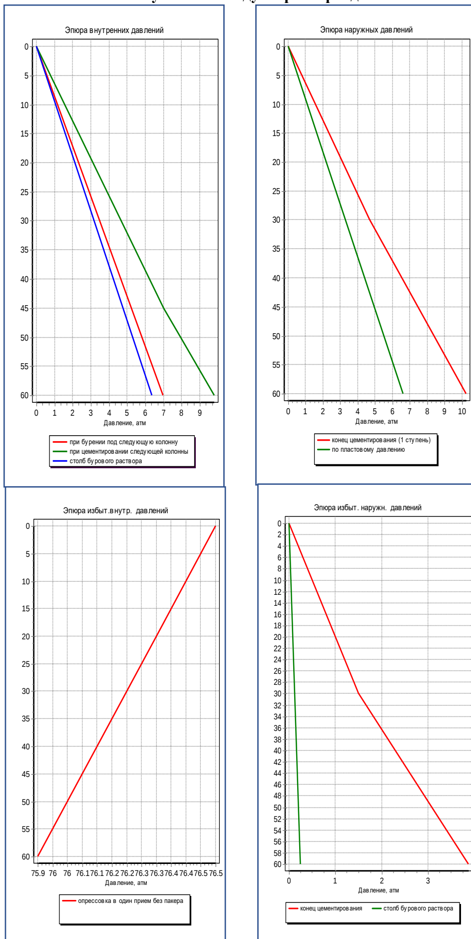
Рисунок 8.2 Кондуктор эпюры давлений
