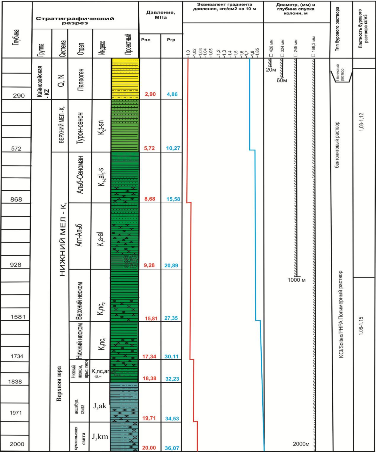
График совмещённых давлений
