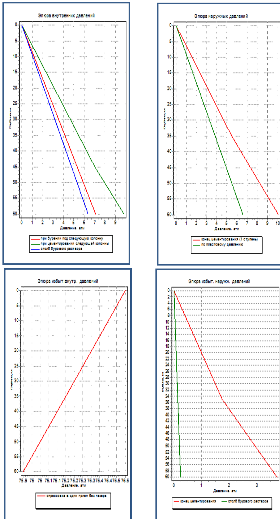
Рисунок 8.2 Кондуктор эпюры давлений
