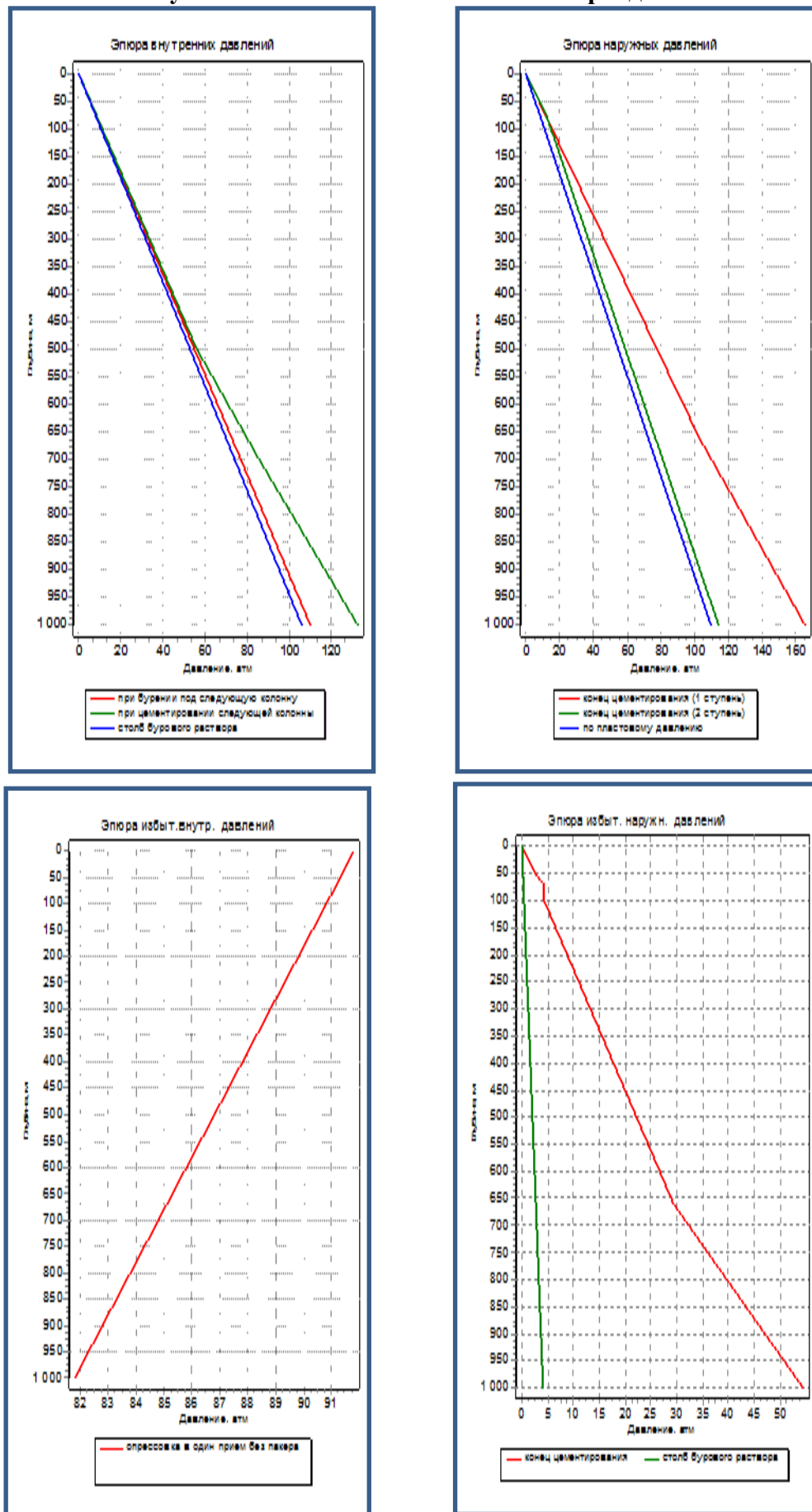
Рисунок 8.3 Техническая колонна эпюры давлений
