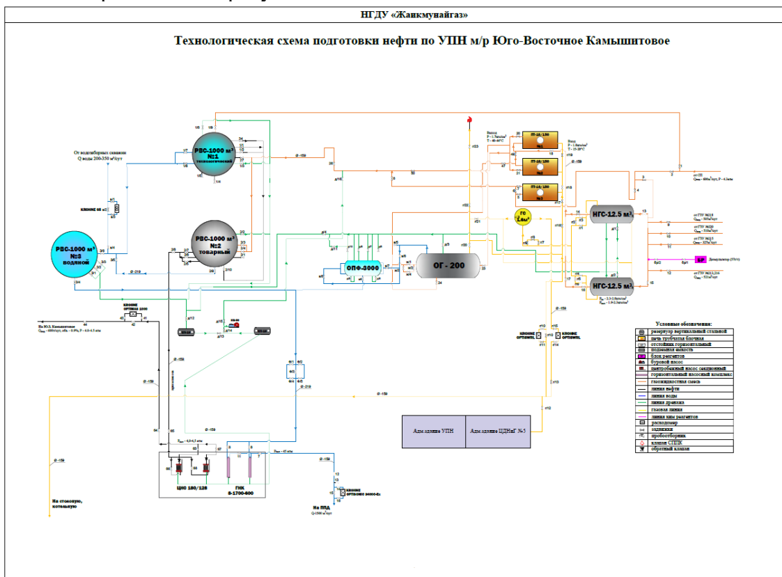
Рисунок 8.9 – Технологическая схема УПН месторождения Юго-Восточное Камышитовое
