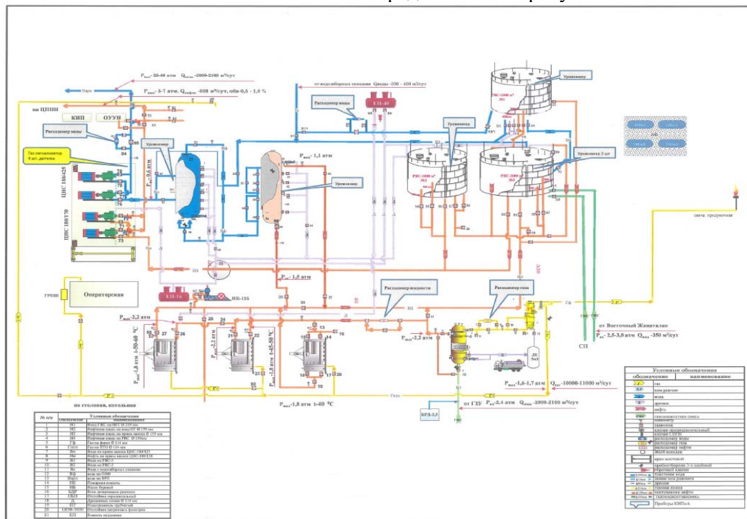
Рисунок 8.13 - Принципиальная схема УПН Жанаталап
