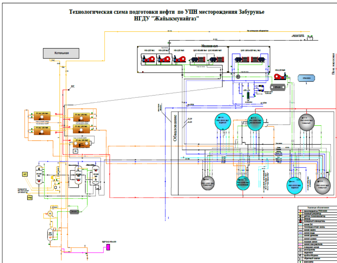
Рисунок 8.16 Технологическая схема пункта подготовки нефти УПН
