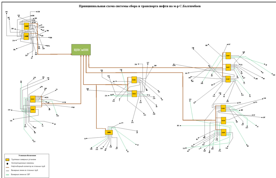
Рисунок 8.2 - Принципиальная схема системы сбора и транспорта нефти месторождения С.Балгимбаев
