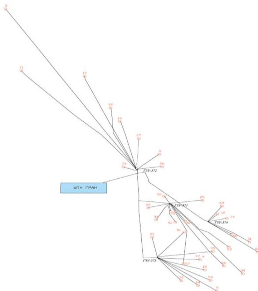
Рисунок 8.14 Принципиальная схема системы сбора скважинной продукции месторождения Гран
