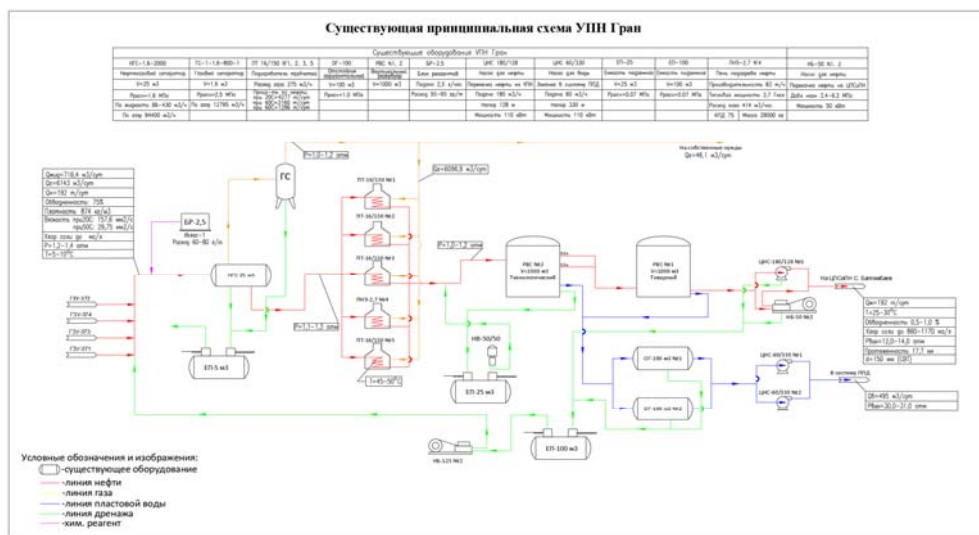
Рисунок 8.15 Существующая принципиальная схема УПН Гран
