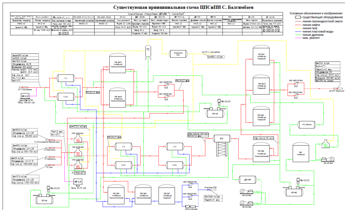
Рис. 8.3 - Существующая принципиальная схема ЦПСиПН С.Балгимбаев Установка подготовки газа (УПГ) на месторождении С. Балгимбаева
