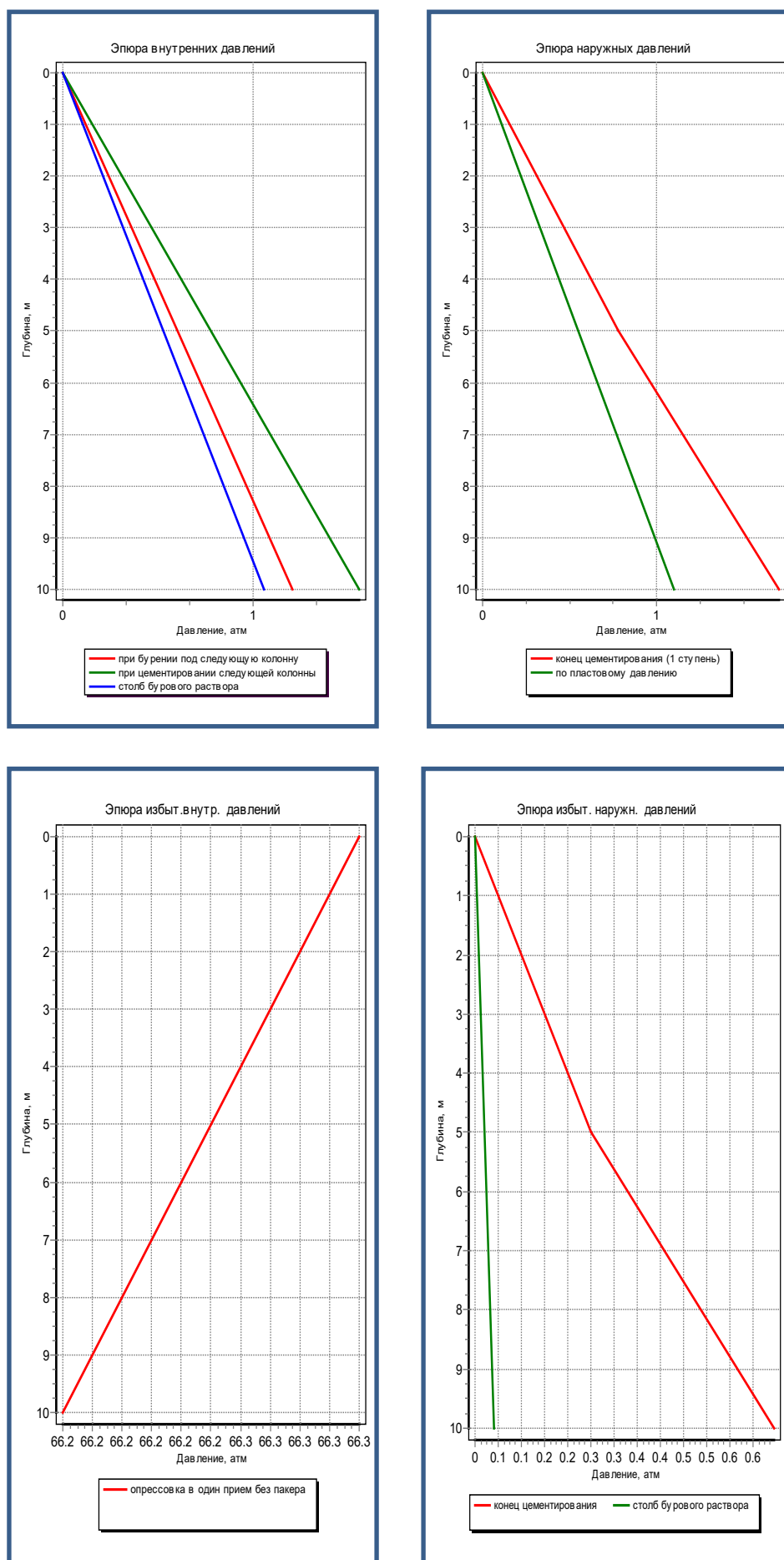
РИСУНОК 8.2 НАПРАВЛЕНИЕ ЭПЮРЫ ДАВЛЕНИЙ
