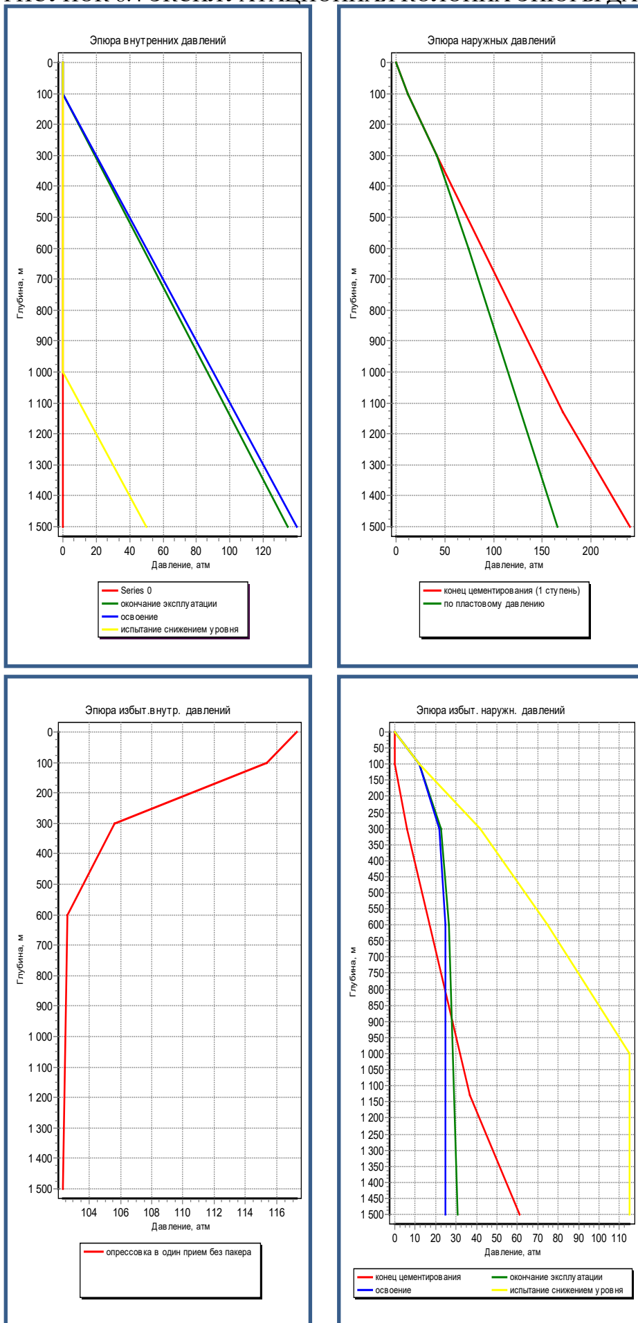
РИСУНОК 8.4 ЭКСПЛУАТАЦИОННАЯ КОЛОННА ЭПЮРЫ ДАВЛЕНИЙ
