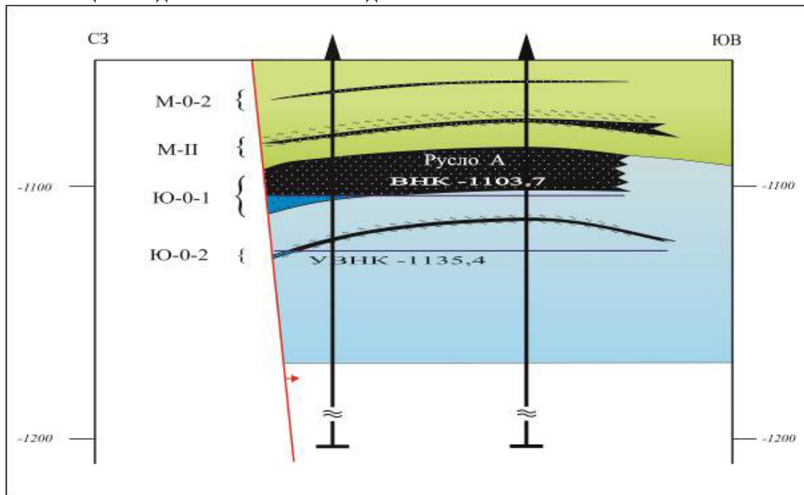
Рис. 1.2 Распределение продуктивных горизонтов по разрезу
