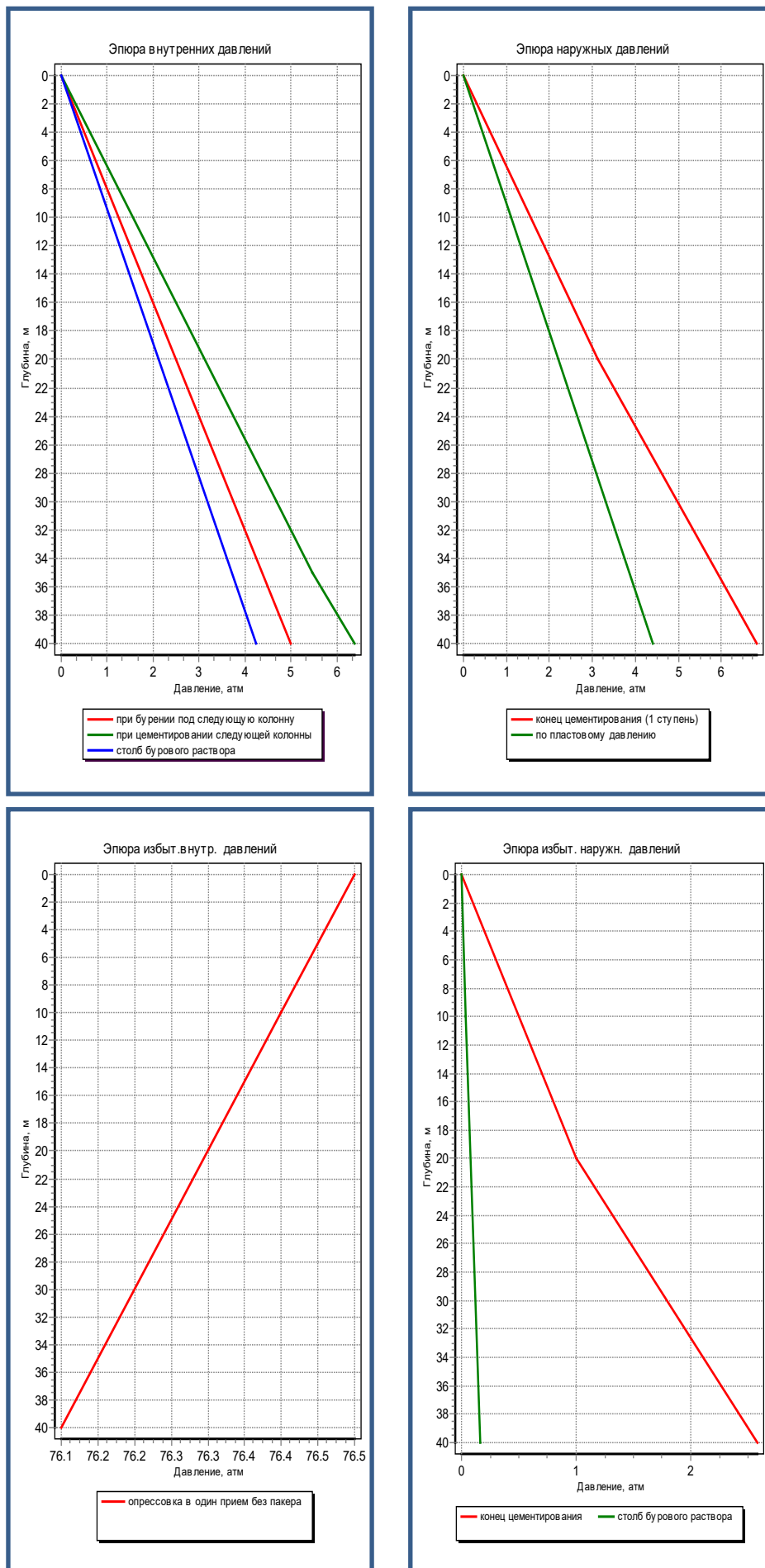
РИСУНОК 8.2 КОНДУКТОР ЭПЮРЫ ДАВЛЕНИЙ
