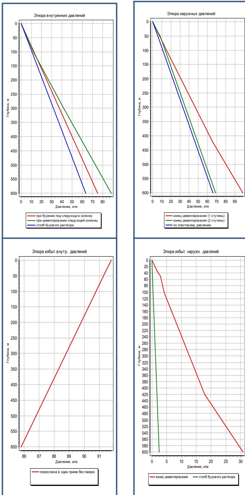
РИСУНОК 8.3 ТЕХНИЧЕСКАЯ КОЛОННА ЭПЮРЫ ДАВЛЕНИЙ
