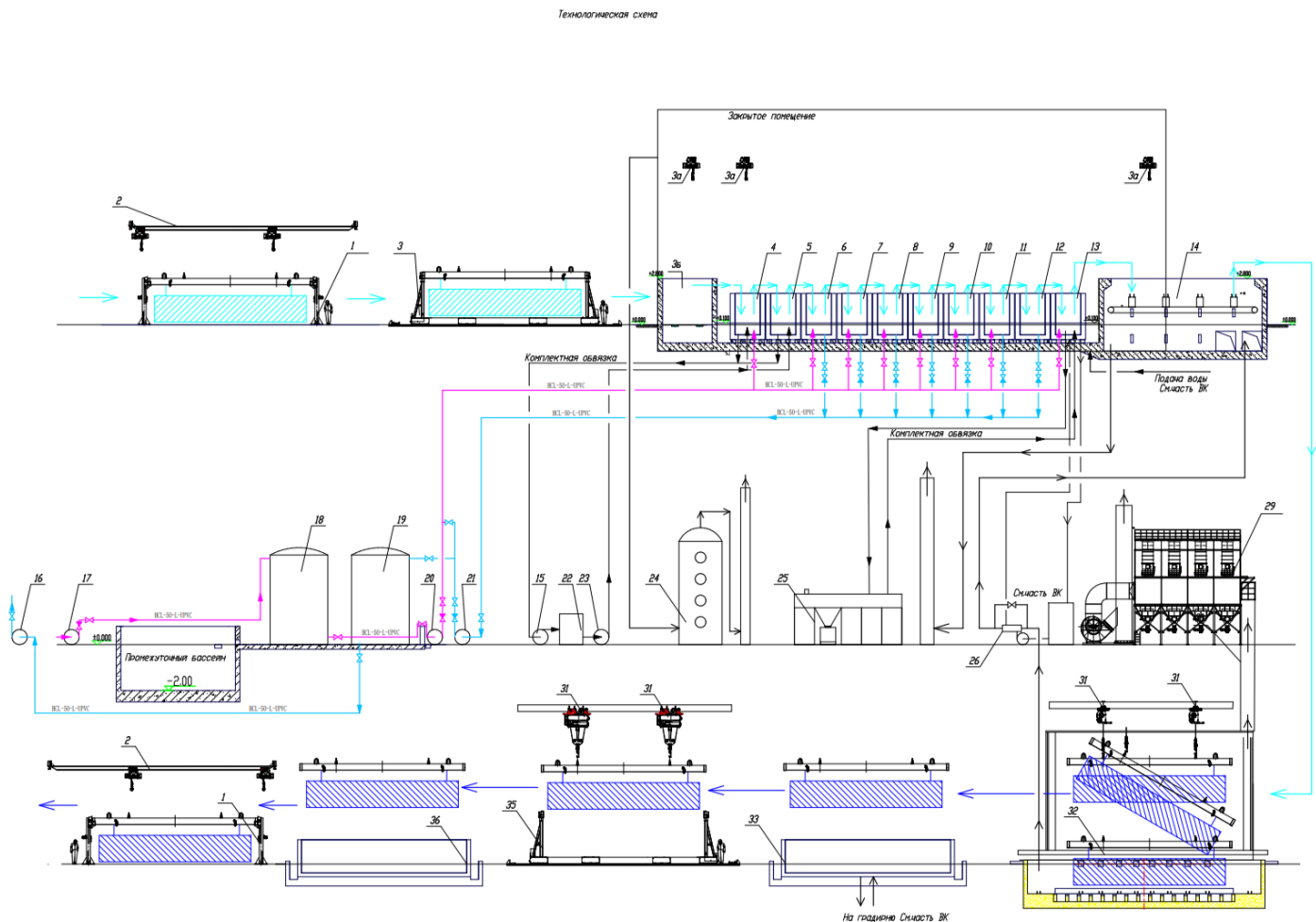
Рисунок 1.1 – техноложическая схема
