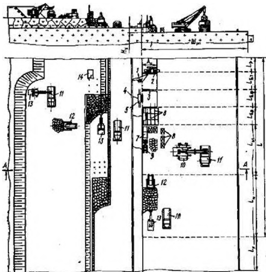
Рис. 2. Слойная панельно-пологая технологическая схема добычи гранитных блоков при термоклинном способе подготовки их к выемке и разработке массивов:
