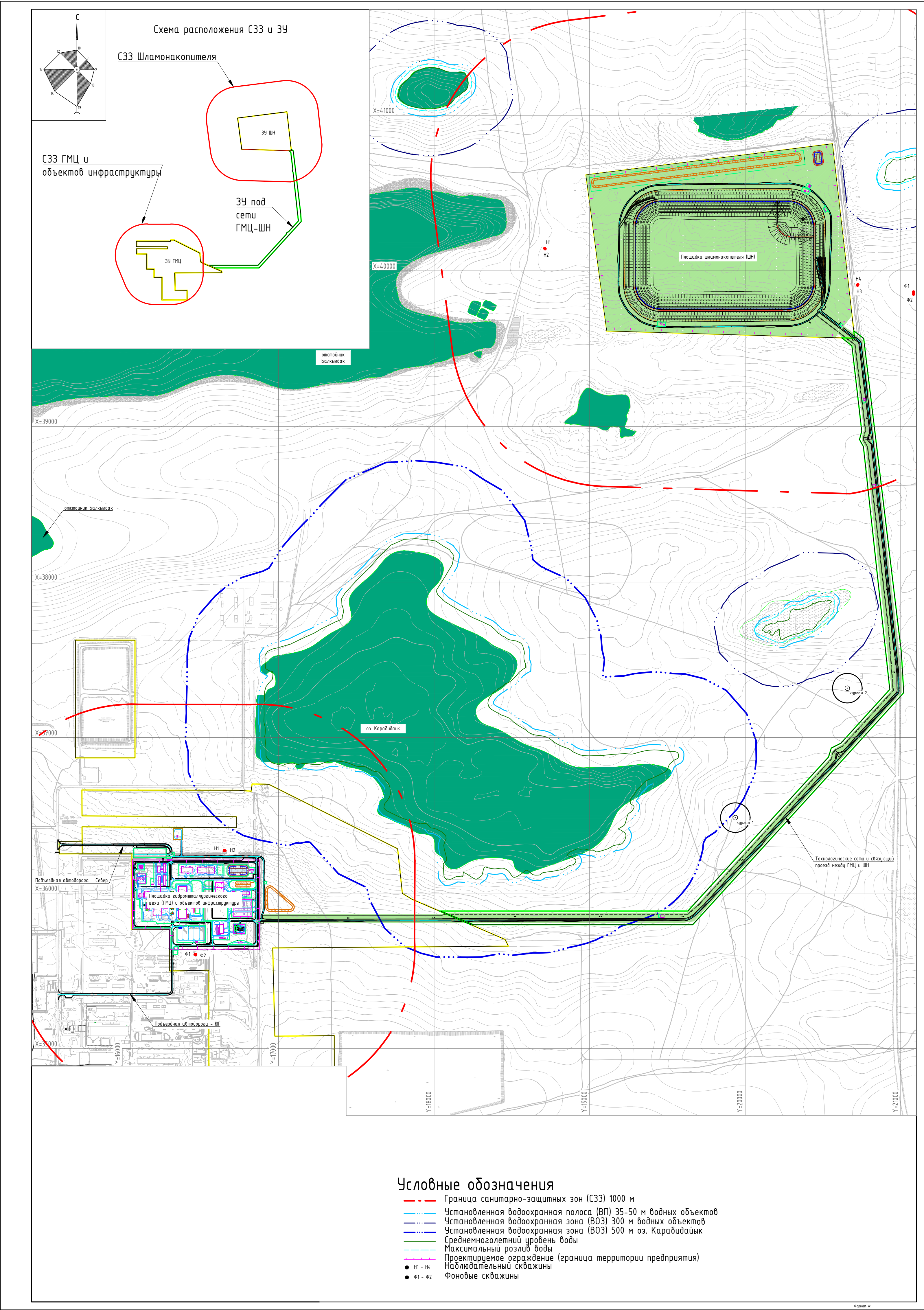
Карта-схема с указанием ВЗ и ВП водных объектов, наблюдательных и фоновых скважин для контроля качества подземных вод
