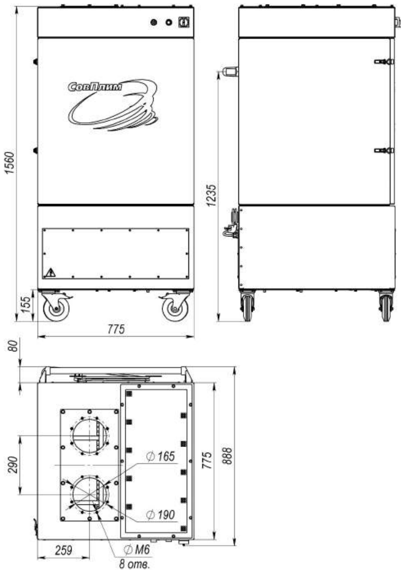
Рисунок А.2 – Габаритные и присоединительные размеры моделей фильтра ПМСФ-6-2х160, ПМСФ-6-2х160-К
