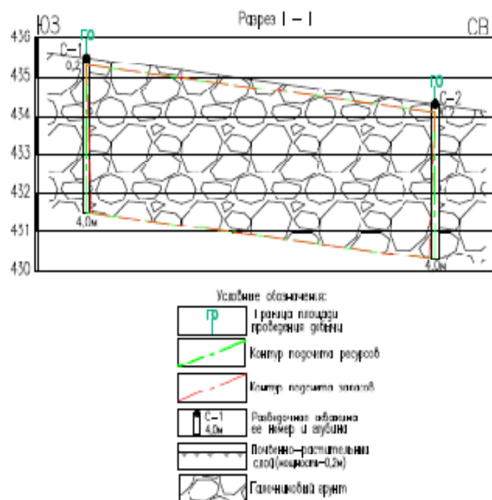
Рис. 2.5 Схема геологического строения участка №25-W
