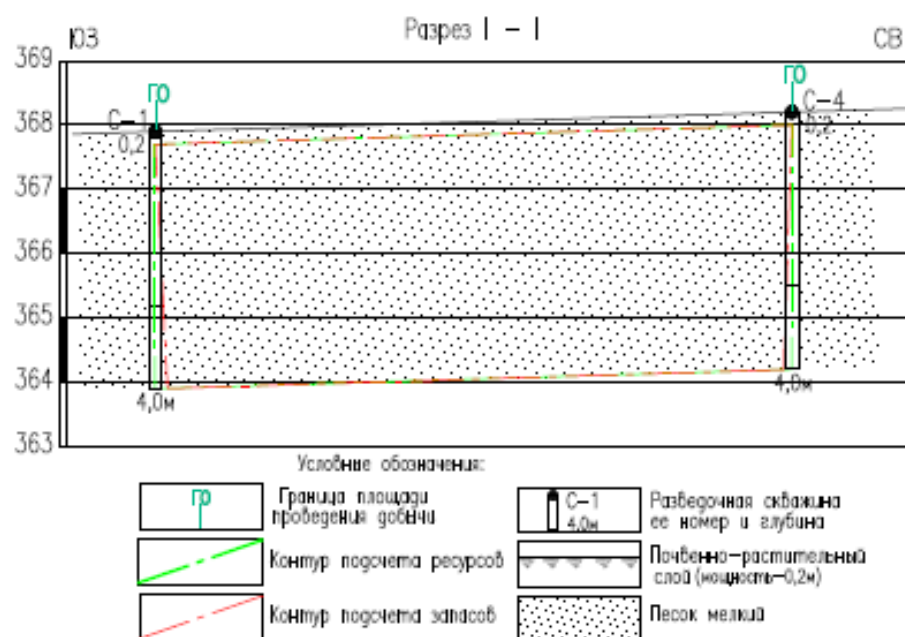
Рис. 2.6 Схема геологического строения участка №26-W
