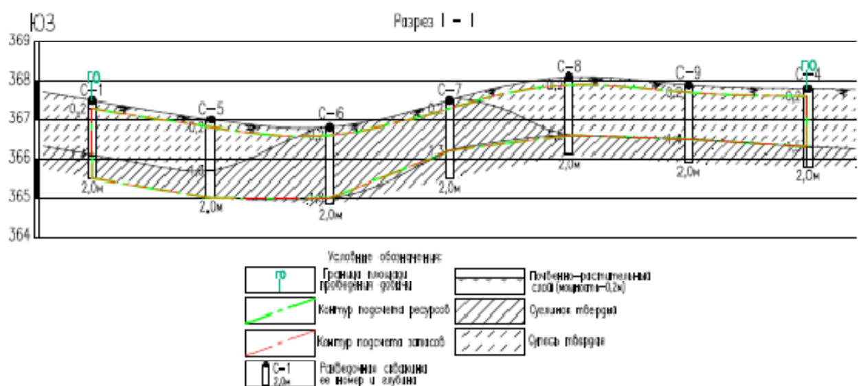
Рис. 2.7 Схема геологического строения участка №27-W
