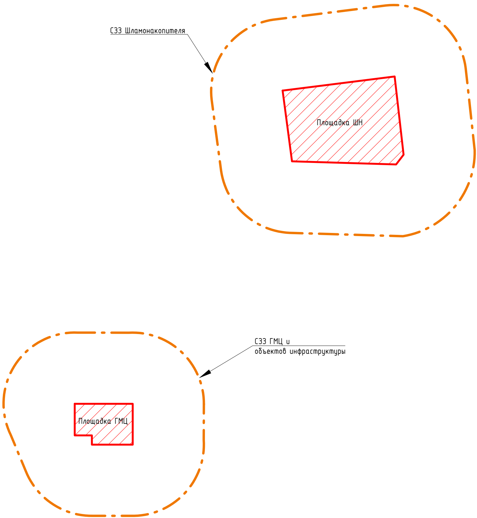
Схема расположения СЗЗ
