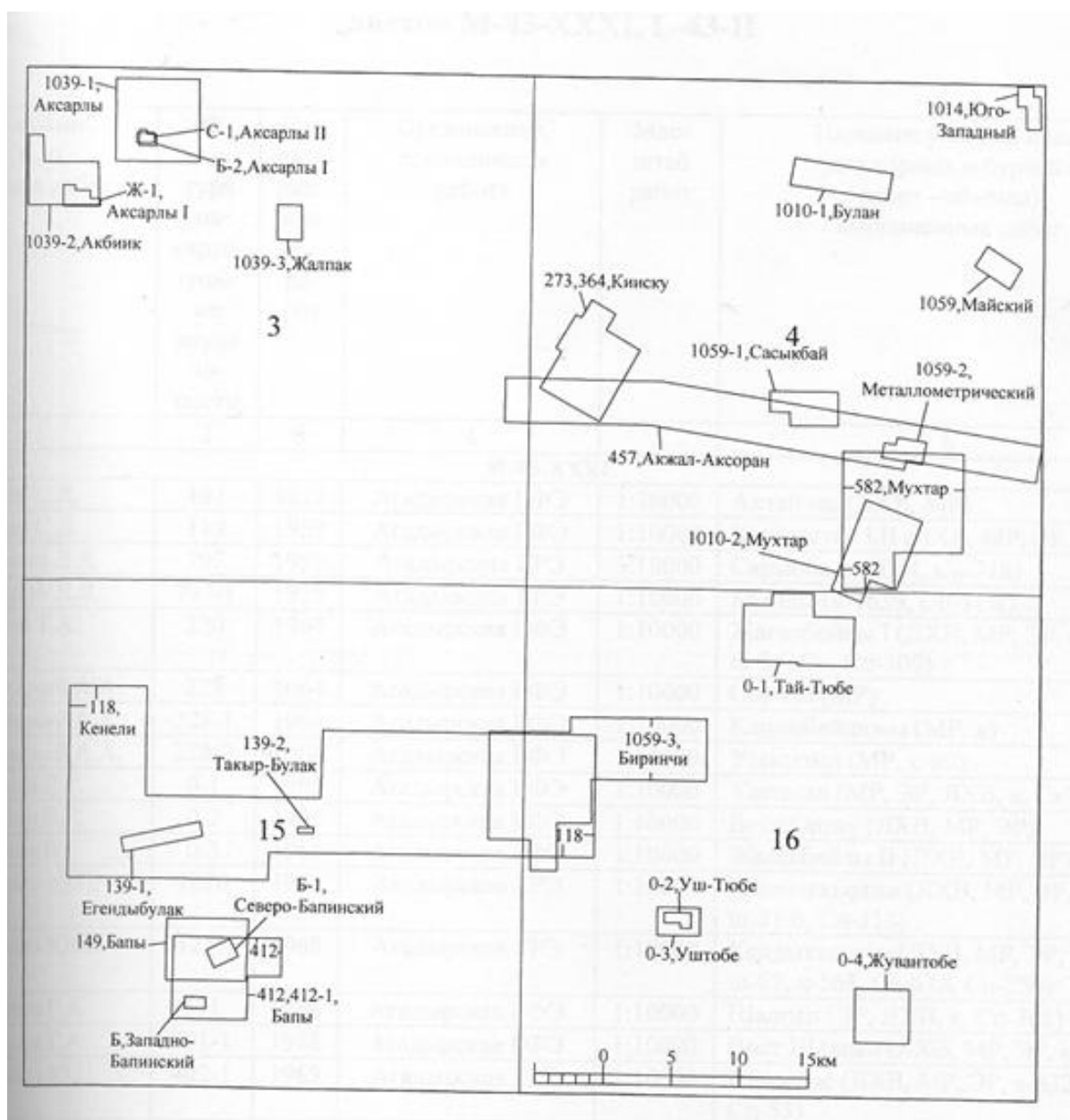
Рис.3 Картограмма геолого-геофизической изученности листа L-43-II.
