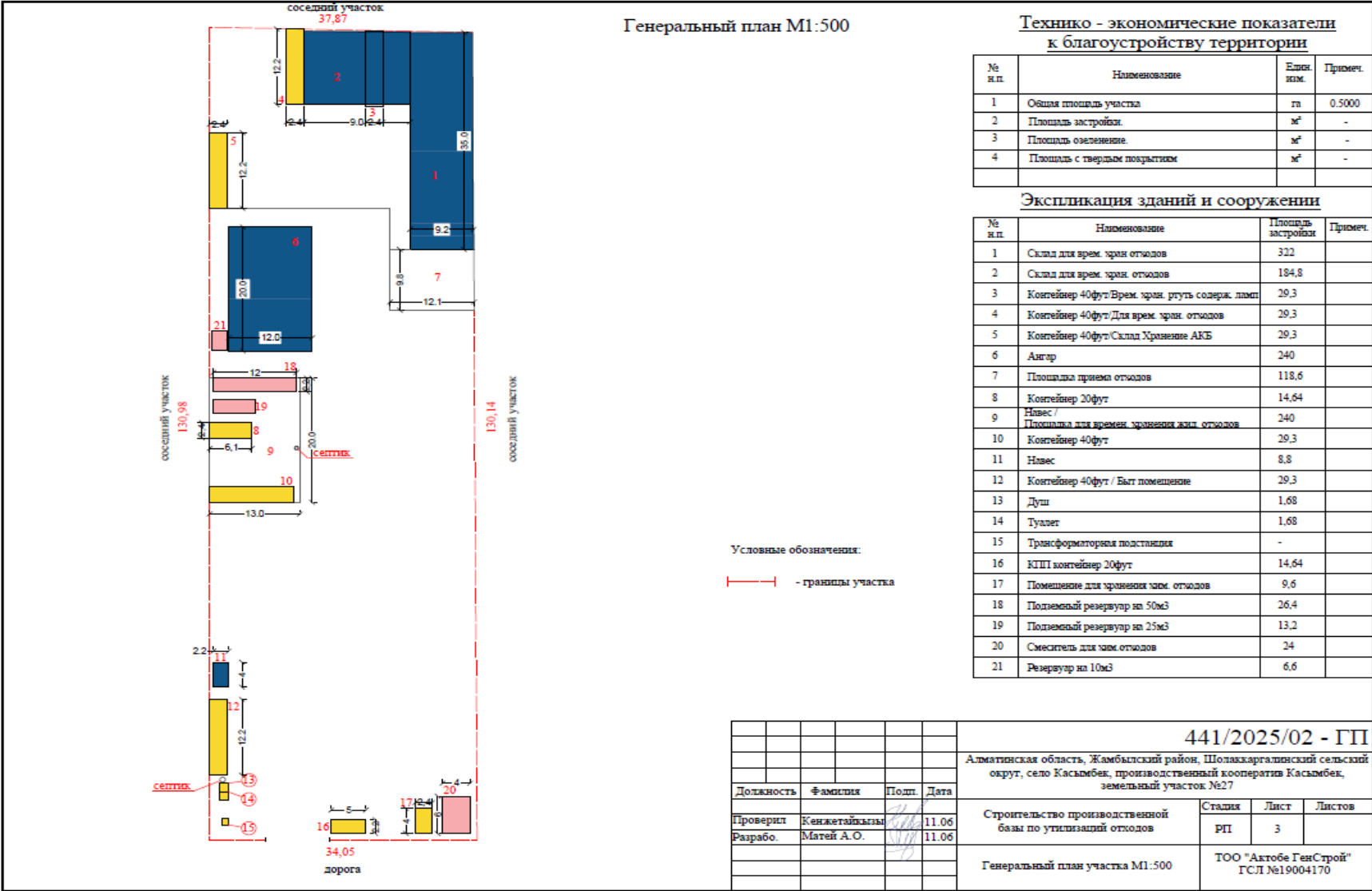
Рис 1.2 – Генеральный план расположения объекта
