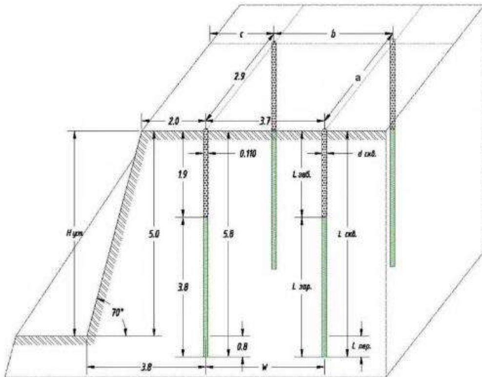
Рисунок 1.4 Параметры конструкции скважинного заряда на рудных уступах
