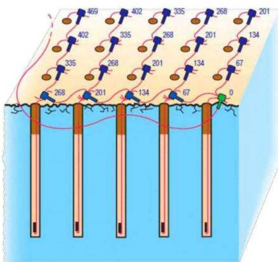
Рисунок 1.5 Схема монтажа взрывной сети при производстве буровзрывных
