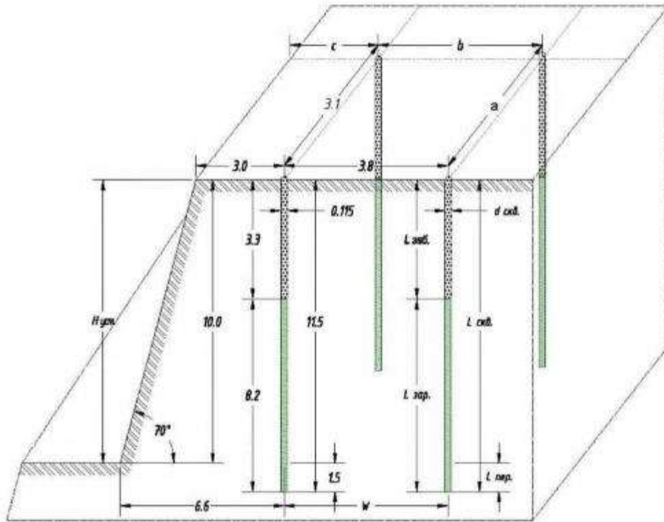
Рисунок 1.3 Параметры конструкции скважинного заряда на вскрывше
