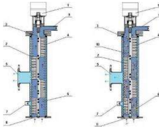
Рисунок 1.7 Процесс очистки в фильтрах ССФ
