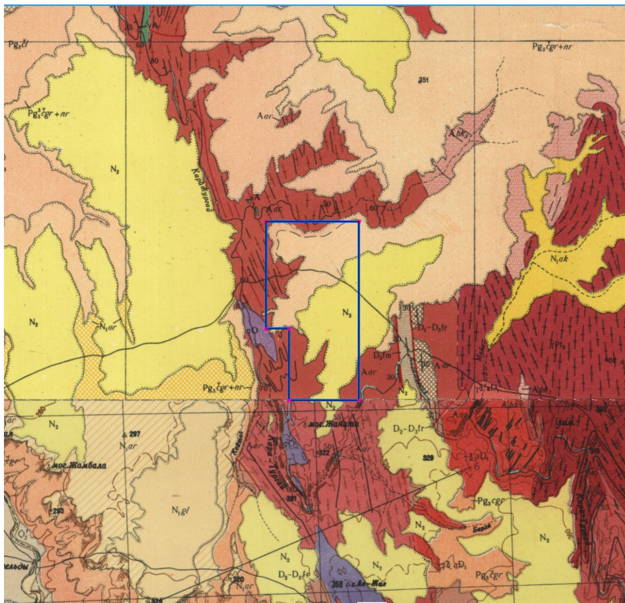
Рис. 4 Геологическая карта района работ
