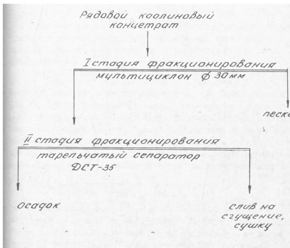
Рис 4.2 Схема получения тонкодисперсного каолина
