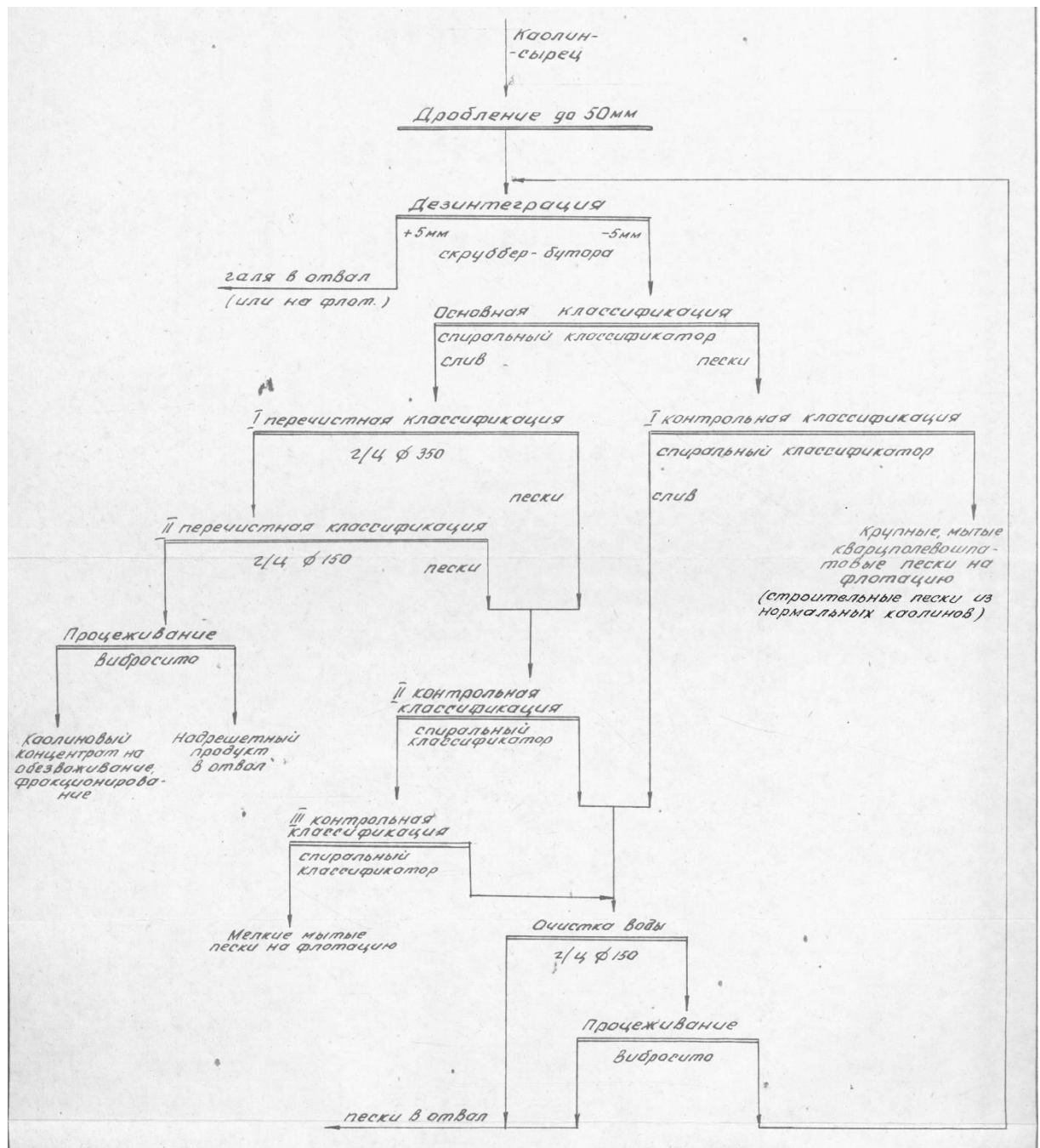
Рис 4.1 Схема обогащения каолина
