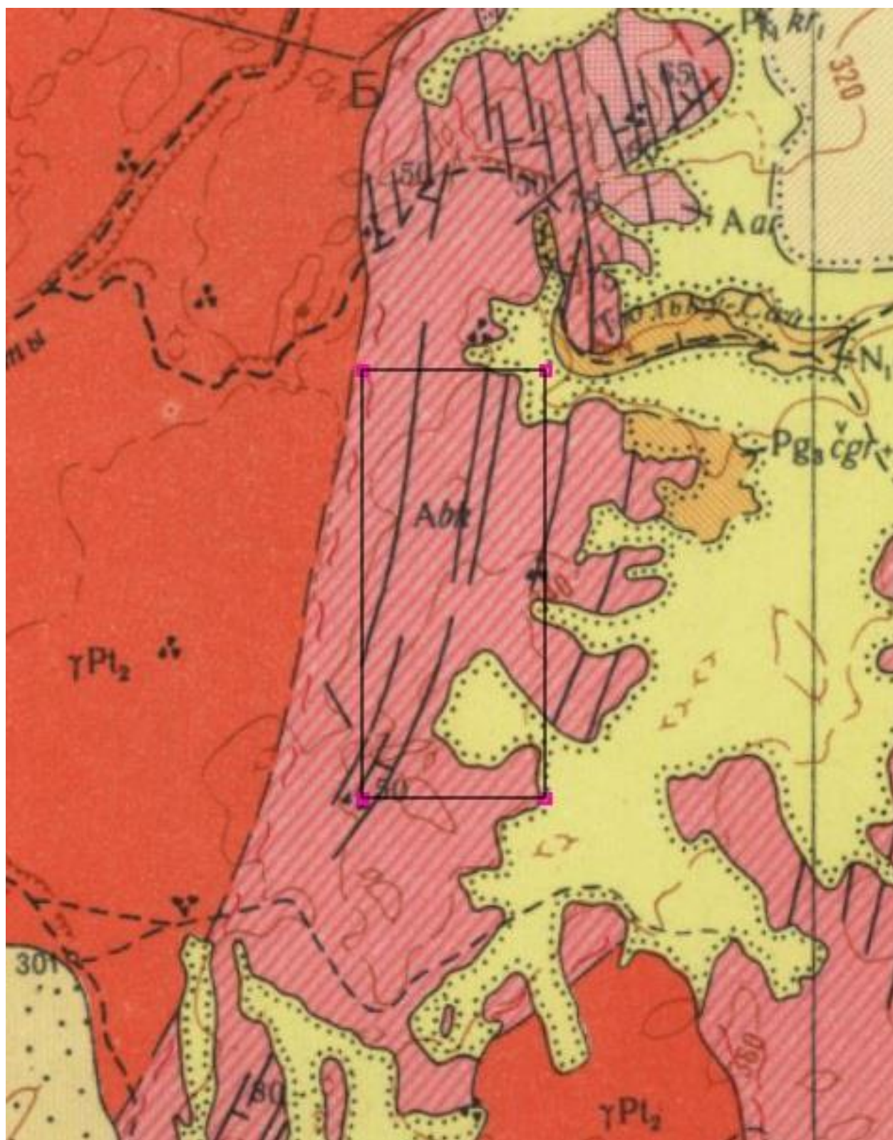
Рис. 4 Геологическая карта района работ
