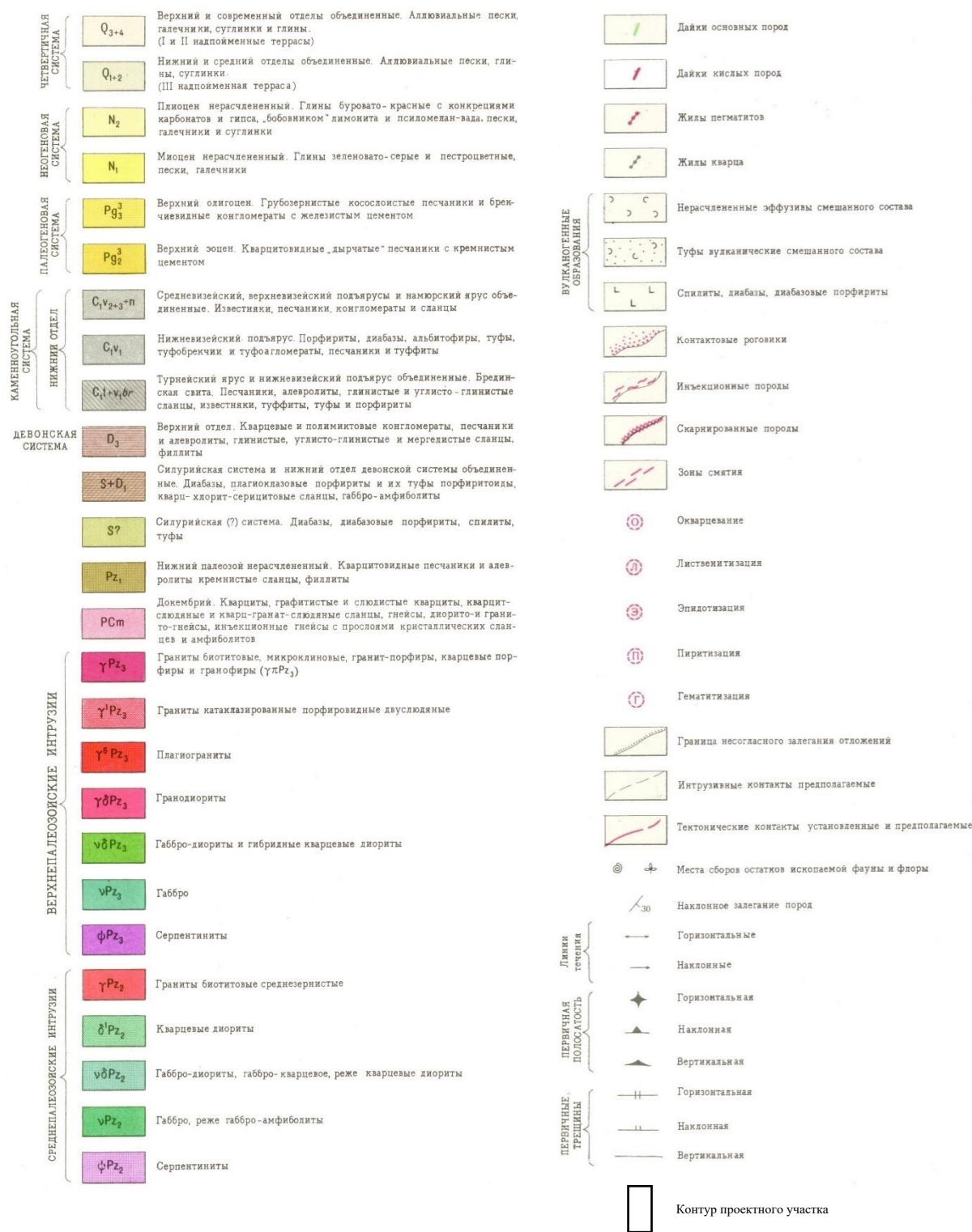
Рис. 5. Условные обозначения к геологической карте района работ
