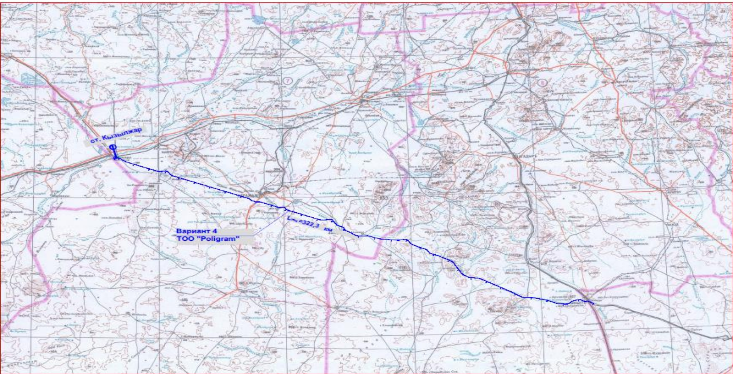
2-сурет. Теміржол трассасының №4 нұсқасы
