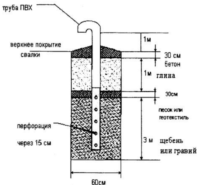
Рисунок 6 – Схема газовыпуска при устройстве системы сбора газа
