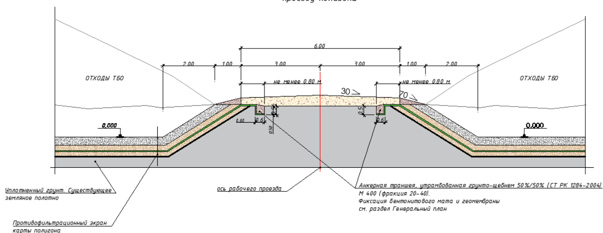
Поперечное сечение по картам складирования и рабочему проезду полигона
