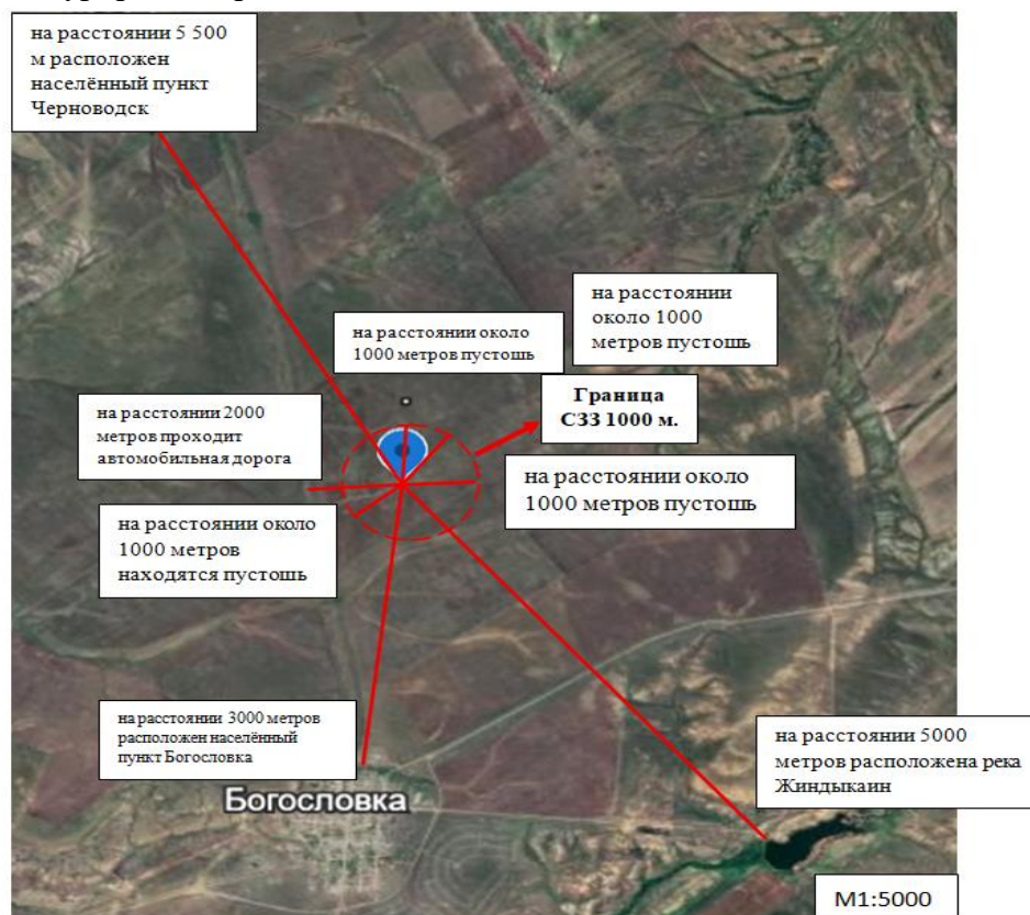
Рис.1 Ситуационная план-схема
