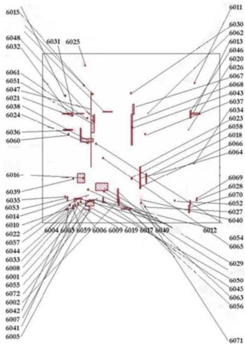
Рисунок 2.2 Ситуационная карта–схема с нанесением источников загрязнения
