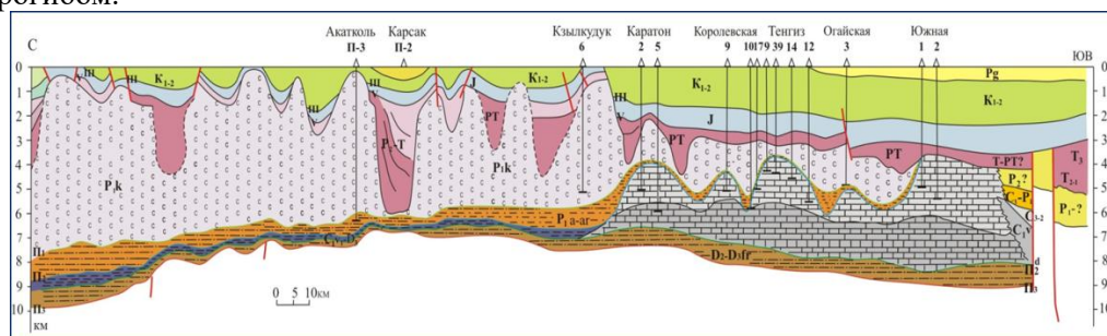
Рис. 5. Геологический разрез по линии Каратон-Тенгиз-Южная (По В.М. Пилифосову, Э.С. Воцалевскому, 2000).
