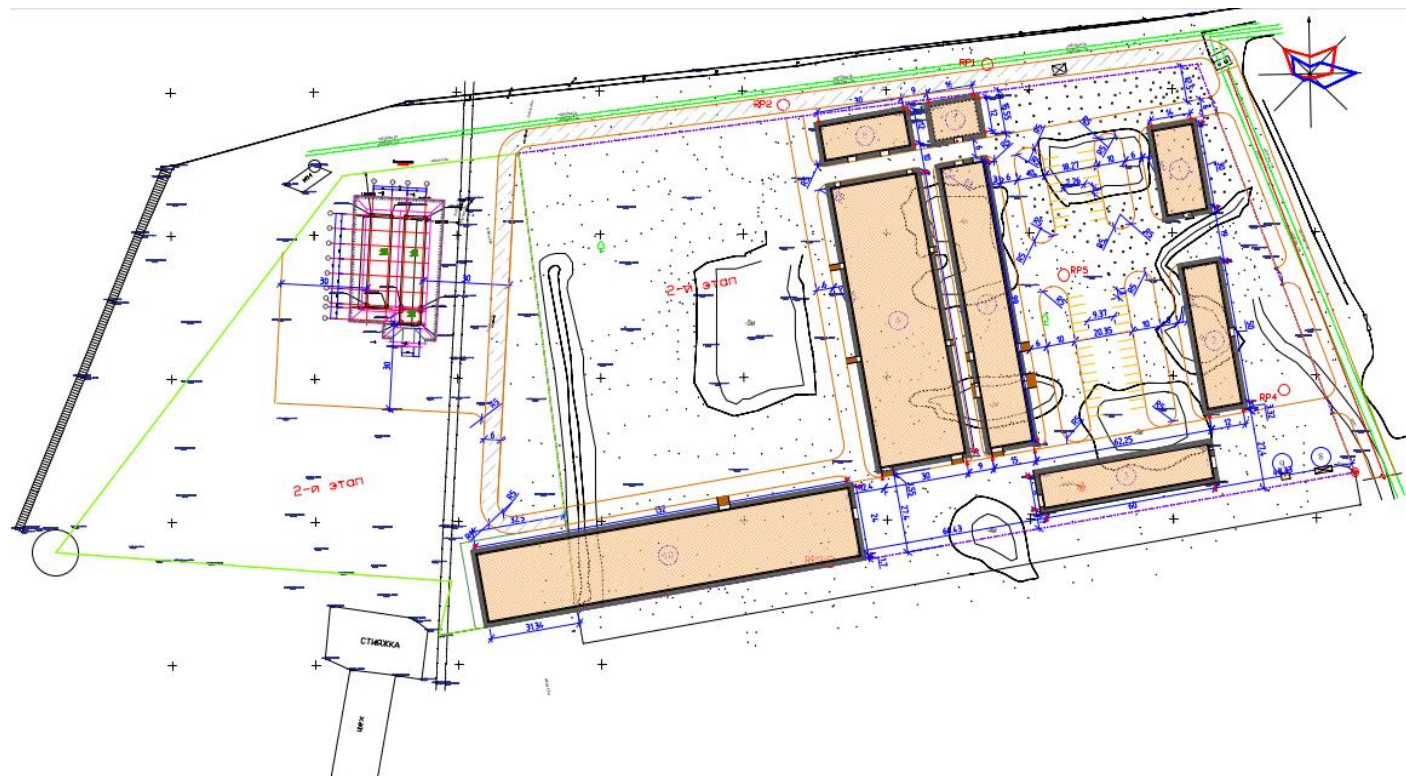
Рис. 10- Разбивочный план
