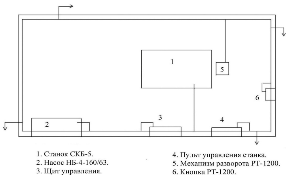
Рис. 1.6.8. Схема защитного заземления на буровом агрегате
