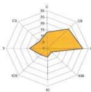
Рис. 1.2.1 – Роза ветров
