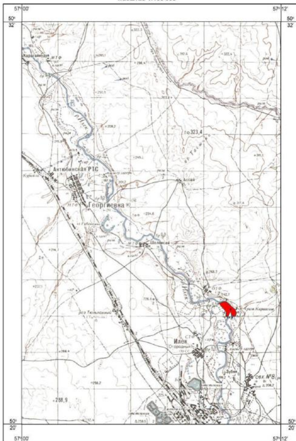
Контур Горного отвода с номерами угловых точек (Северный участок Георгиевского месторождения)
