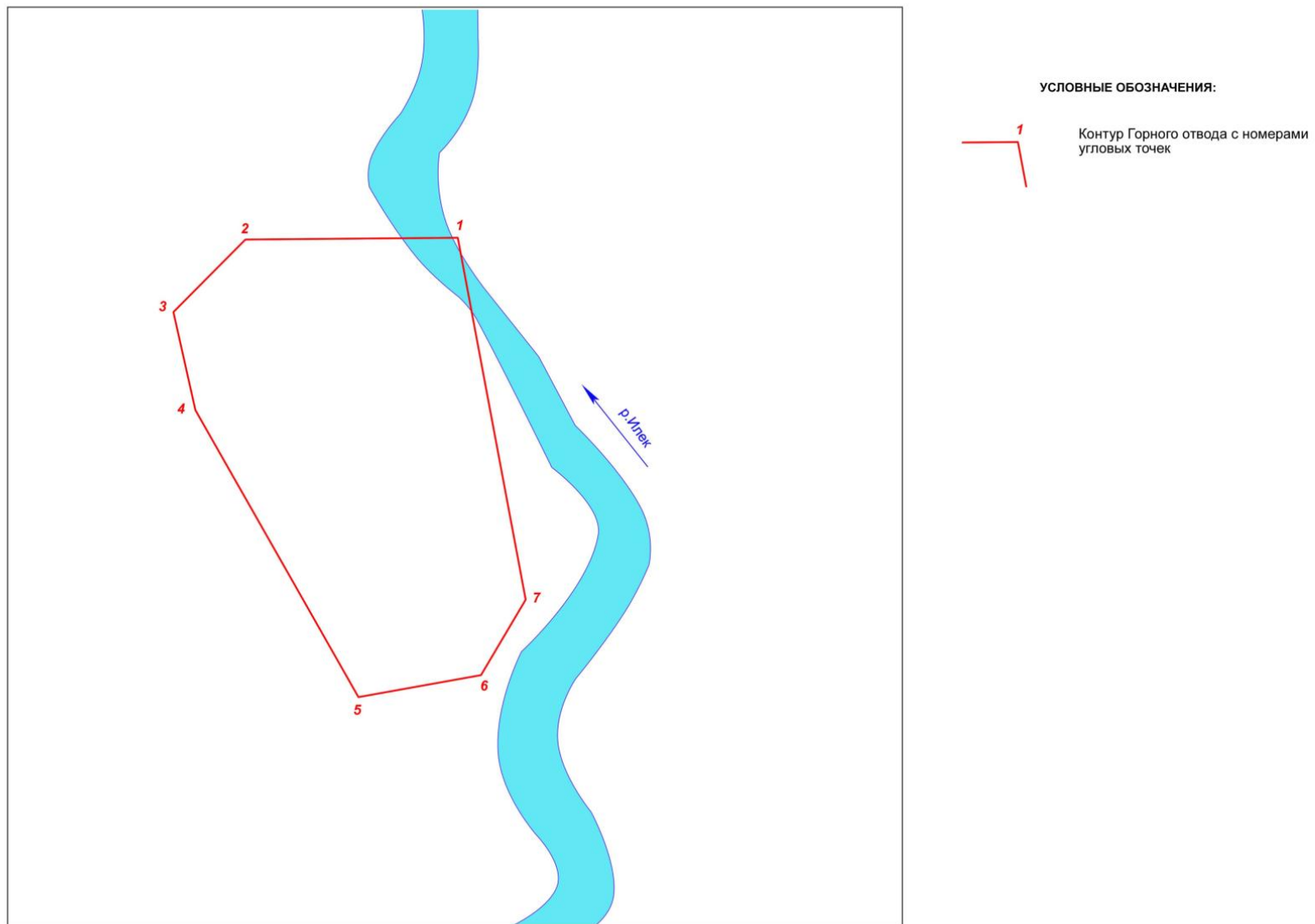
Рис.3. Ситуационный план на начало разработки карьера. Масштаб 1:5 000
